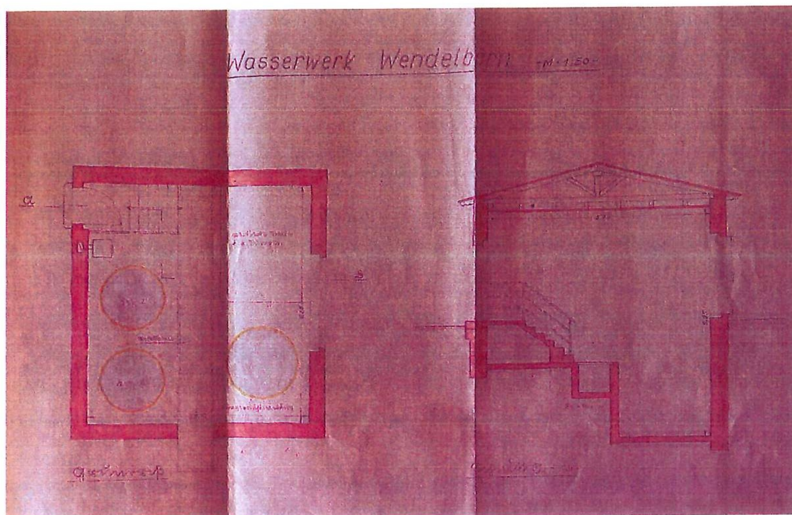
il. 27 Projekt oczyszczalni wody, 1941, Archiwum Państwowe w Wrocławiu.
