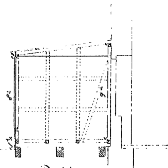
Profil
