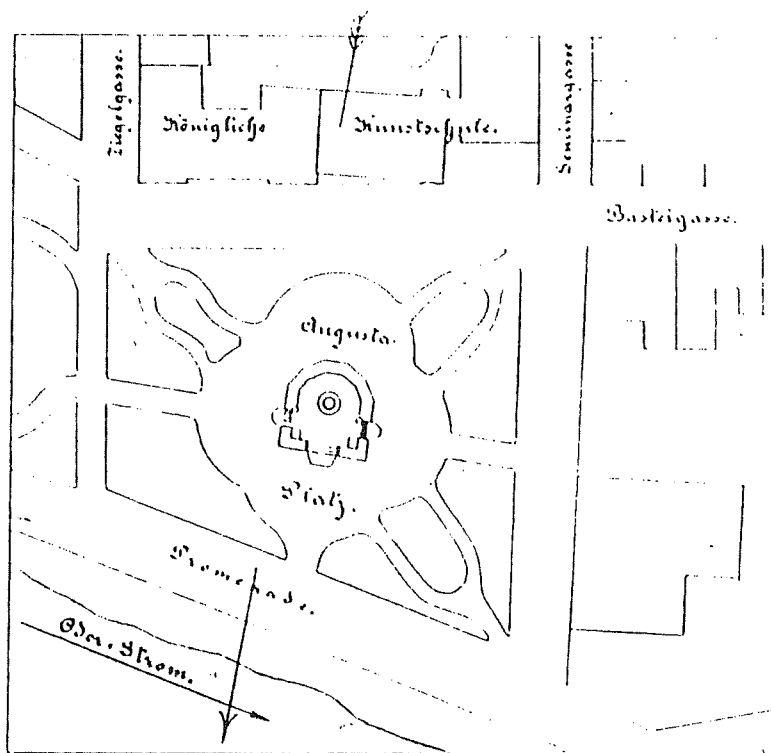
Lageplan.
