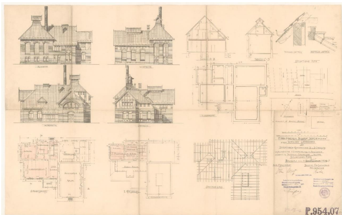
Il. 3 Gazownia. Murowane nakrycie dachu w systemie Schürmann, 1907, podpisano: Urząd Budowlany: Karbe, Magistrat: Wirtz (plik 127572). Archiwum Budowlane Wrocław, teczka 3455.
