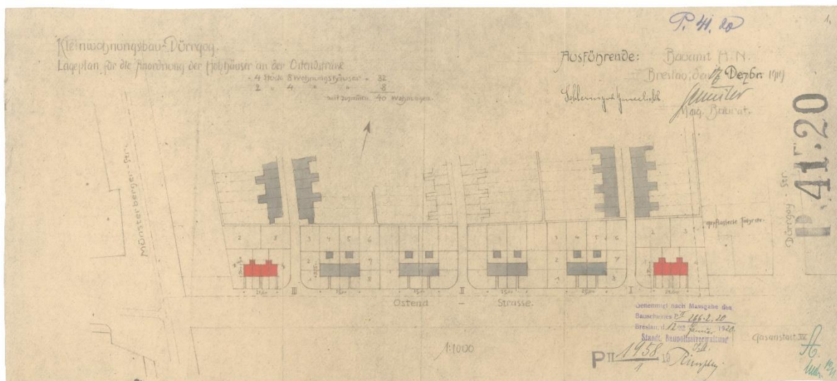
Il. 23 Ul. Gazowa. Plan sytuacyjny budynków po północnej stronie ulicy, 1919, podpisano: Radca budowlany magistratu: ? (plik 157343). Archiwum Budowlane Wrocław, teczka 3458.
