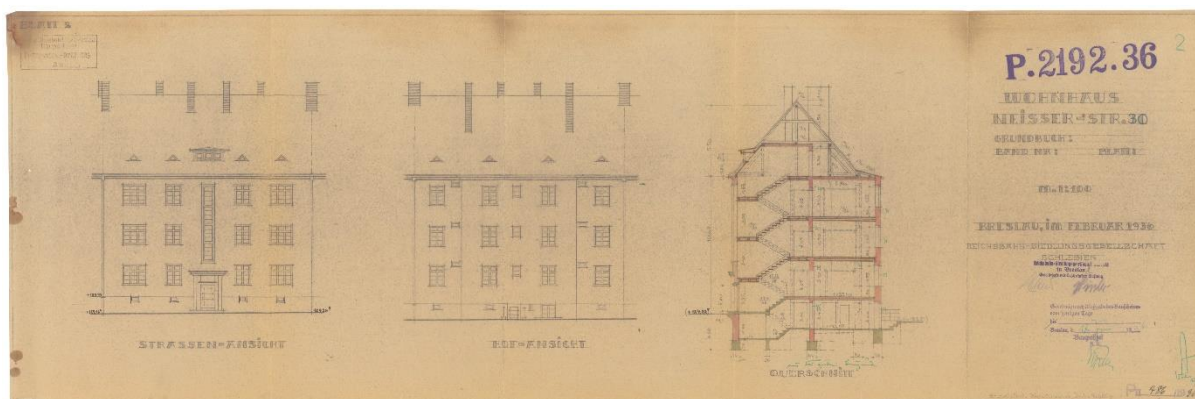
Il. 101 Ul. Nyska. Elewacje i przekrój budynku nr 30, 1936, Inwestor: Reichsbahn-Siedlungsgesellschaft Schlesien in Breslau (plik 103361). Archiwum Budowlane Wrocław, teczka 3090.
