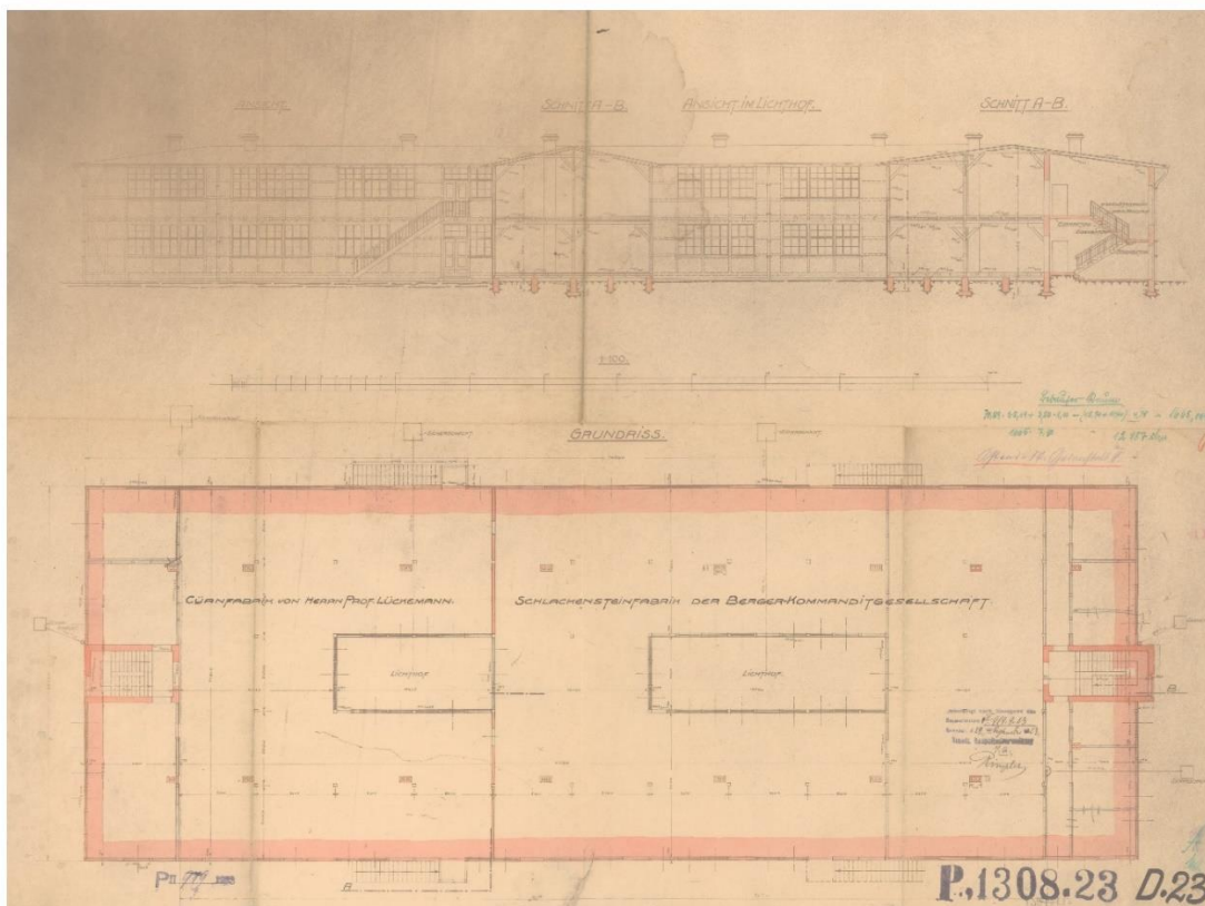
Il. 12 Gazownia. Szkic budowy fabryki cijanu i fabryki bloczków żużlobetonowych, 1923, podpisano: Magistrat: Rimpler (plik 127599). Archiwum Budowlane Wrocław,teczka 3456.
