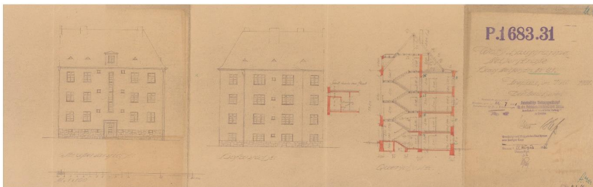
Il. 90 Ul. Nyska. Elewacje i przekroje budynku 21, 1931, Inwestor: Gemeinnützige Siedlungsgesellschaft für den Reichsbahndirektionsbezirk Breslau (plik 103287). Archiwum Budowlane Wrocław, teczka 3089.
