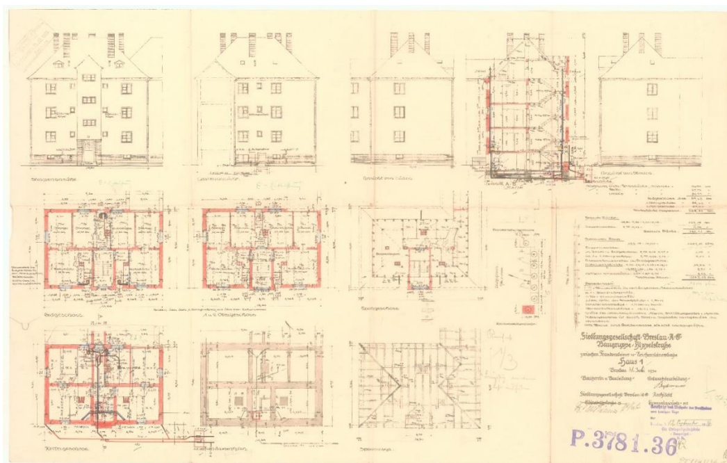
Il. 55 Ul. Złotostocka. Budynki mieszkalne wznoszone przez Siedlung Gesellschaft Breslau A. G. między Złotostocką a Ząbkowicką, budynek nr 1, 1936, podpisano: Architekt: Busmann (plik 124460). Archiwum Budowlane Wrocław, teczka 3648.
