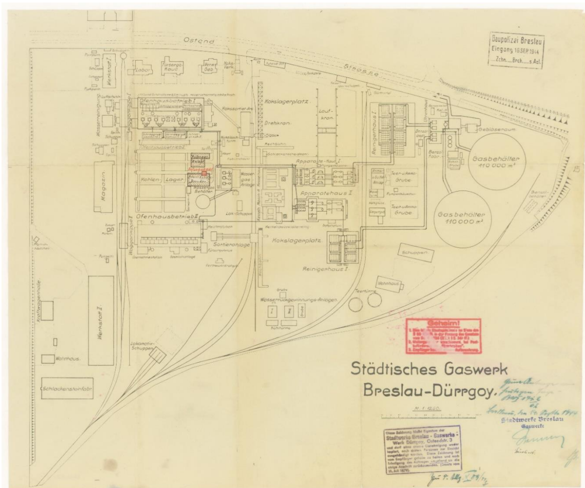
Il. 20 Gazownia. Plan sytuacyjny z funkcjami urządzeń technicznych, 1944 (plik 127516). Archiwum Budowlane Wrocław,teczka 3457.
