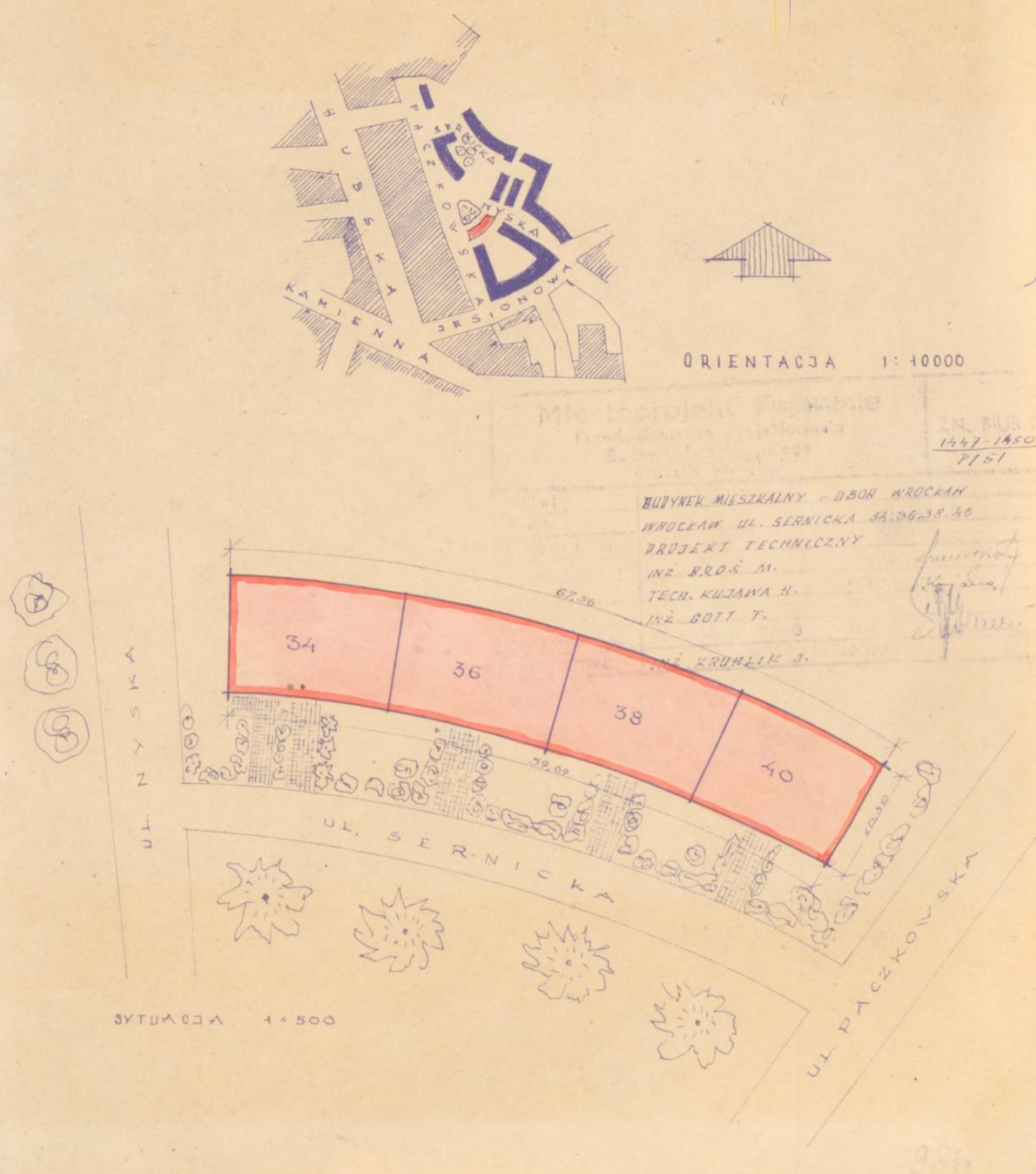
Il. 125 Ul. Sernicka. Plan sytuacyjny i rzut budynków mieszkalny nr 34-40, 1951, Inwestor: Dyrekcja Budowy Osiedli Robotniczych, Projekty techniczne: inż Broś, Kujawa, Kruhlik (plik 30-40 rys.1). Archiwum Budowlane Wrocław, DPL 202
