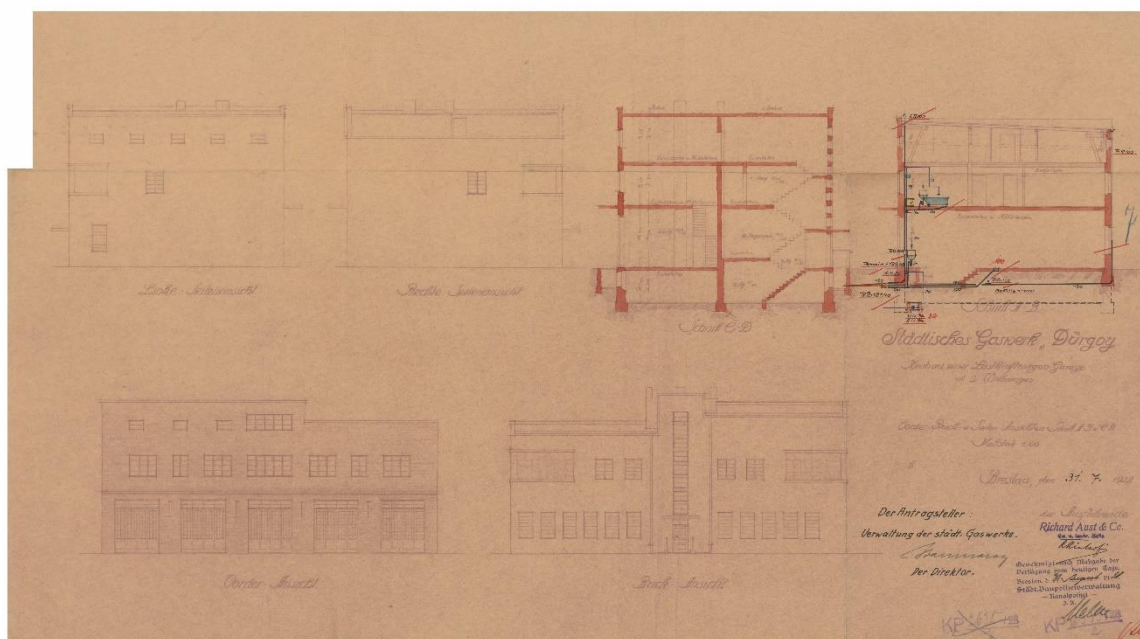
Il. 21 Gazownia. Budowa garażu dla ciężarówek, 1928, podpisano: Wykonawca: Richard Aust (plik 127531). Archiwum Budowlane Wrocław,teczka 3457.
