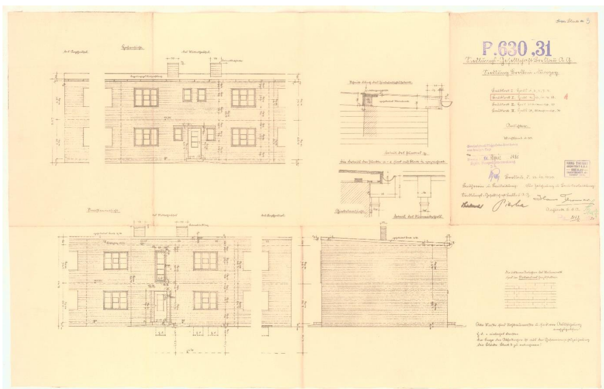
Il. 58 Ul. Złotostocka. Projekt budynku przy ul. Złotostockiej 10, 1931, wznoszonego przez Siedlung Gesellschaft Breslau A. G., podpisano: Architekt: Hans Thomas (plik 124473). Archiwum Budowlane Wrocław,teczka 3648.
