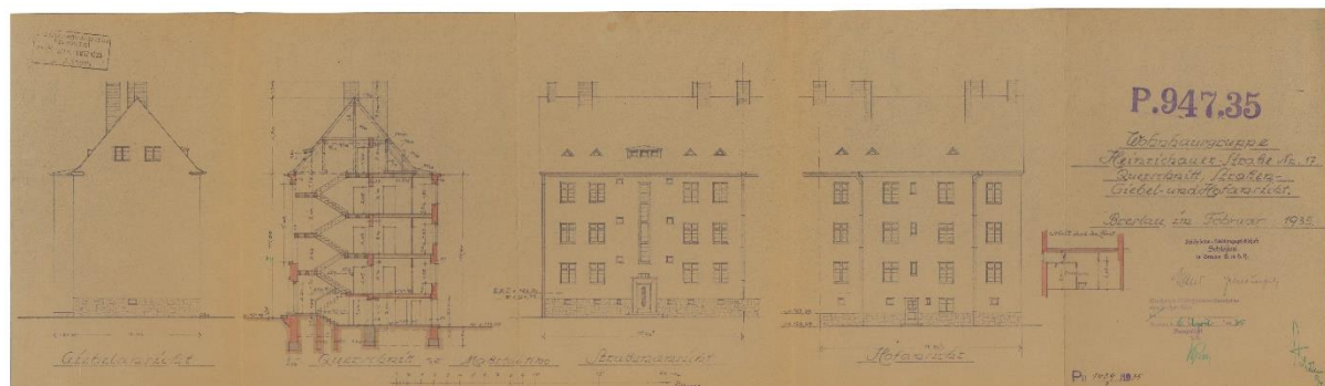
Il. 73 Ul. Henrykowska. Przekroje budynku nr 17, 1935, Inwestor: Reichsbahn-Siedlungsgesellschaft Schlesien in Breslau (plik 103568). Archiwum Budowlane Wrocław,teczka 1712.
