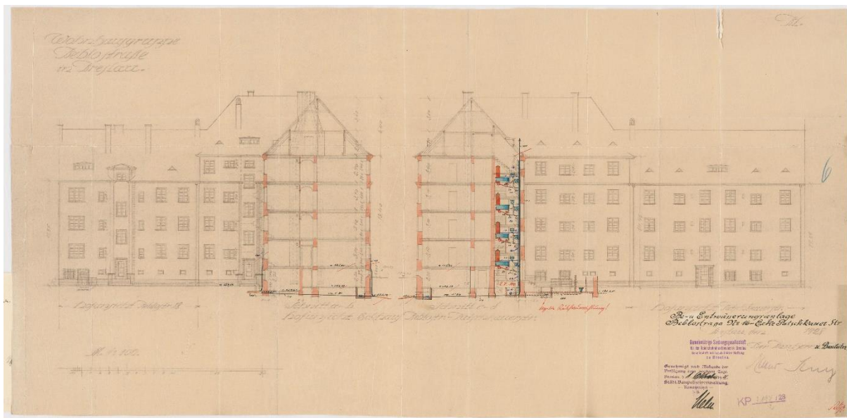
Il. 80 Ul. Jesionowa. Rzuty i widoki elewacji budynków narożnych przy ul. Jesionowej/Paczkowskiej, 1928, Inwestor: Gemeinnützige Siedlungsgesellschaft für den Reichsbahndirektionsbezirk Breslau (plik 97036). Archiwum Budowlane Wrocław, teczka 377.
