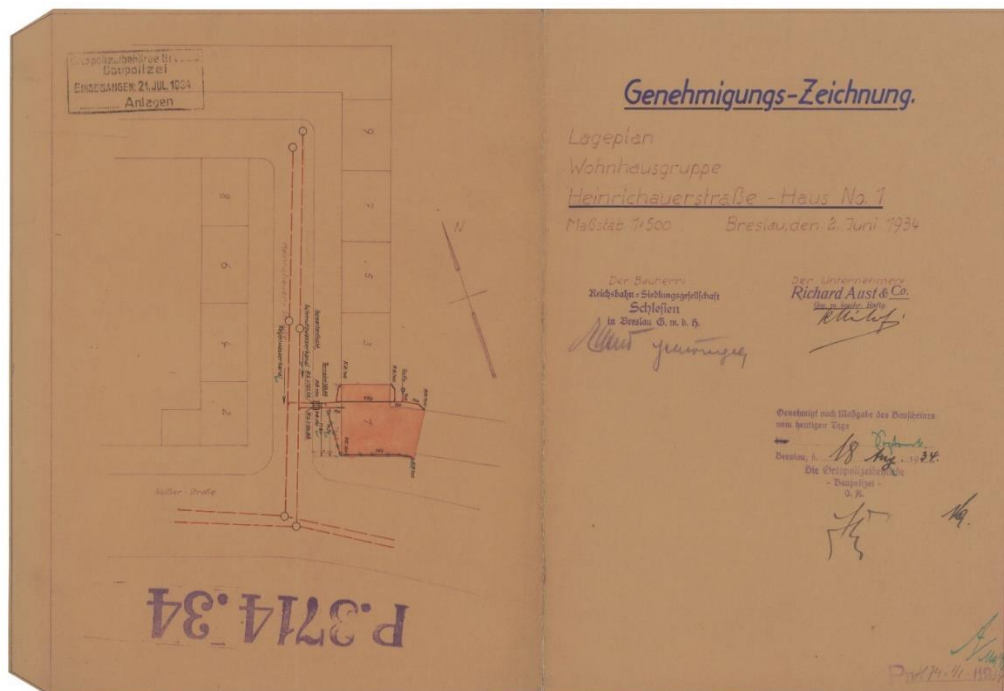
Il. 62 Ul. Henrykowska. Rzut sytuacyjny budynku na narożniku ulic Henrykowskiej i Nyskiej (ul. Henrykowska 1) z rysunkiem podłączenia do sieci wodno-kanalizacyjnej, 1934, Inwestor: Reichsbahn-Siedlungsgesellschaft Schlesien in Breslau, Przedsiębiorca: Richard Aust und Co. (plik 103441). Archiwum Budowlane Wrocław, teczka 1711.
