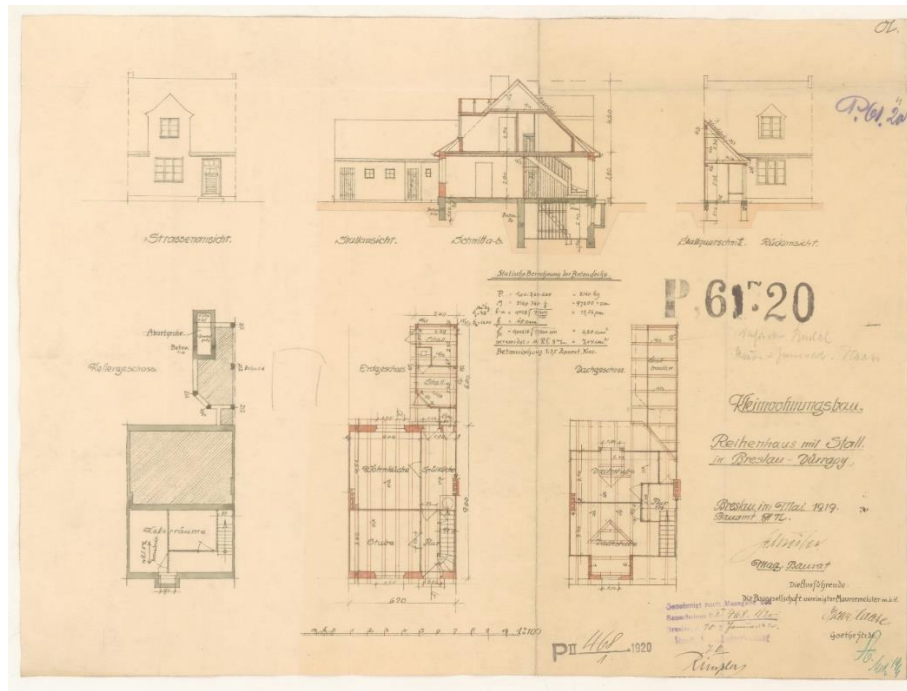
II. 45 Ul. Ząbkowicka. Budynek szeregowy ze stodołą, 1919, podpisano: Wykonawca: Haertel (?) (plik 124608). Archiwum Budowlane Wrocław, teczka 1105.
