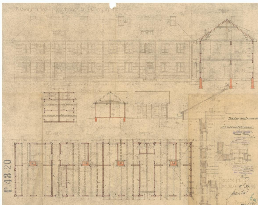
Il. 26 Ul. Gazowa. Plany drewnianego budynku, 1919, podpisano: Architekt: Paul Schreiber, Wykonawca: Przedsiębiorstwo Budowlane: Ernst Isaak (plik 157354). Archiwum Budowlane Wrocław, teczka 3458.
