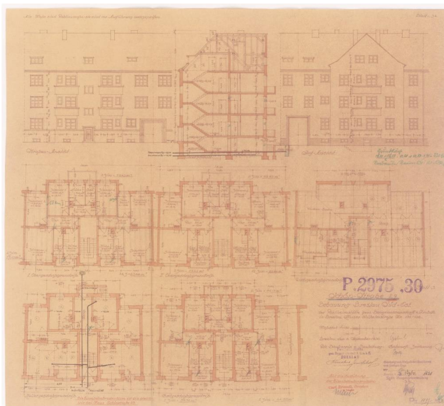
Il. 119 Ul. Piękna. Widok elewacji, przekrój i rzuty budynku nr 27, 1930, Inwestor: Postheimstätte gem. Baugenossenschaft G. m. b. H. Breslau, Architekt: Wolf, Wykonawca: Carl Brandt (plik 103175). Archiwum Budowlane Wrocław, teczka 3980.
