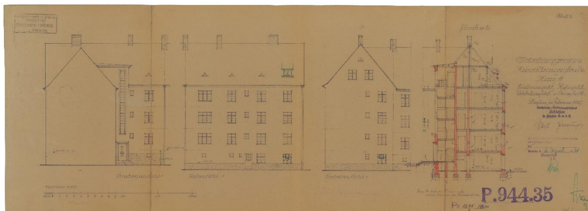
Il. 72 Ul. Henrykowska. Przekroje budynku nr 11, 1935, Inwestor: Reichsbahn-Siedlungsgesellschaft Schlesien in Breslau (plik 103541). Archiwum Budowlane Wrocław,teczka 1712.
