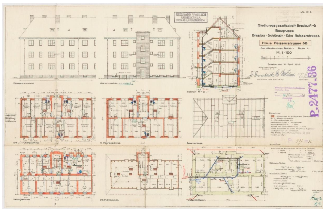
II. 109 Ul. Nyska. Elewacje, przekroje i rzuty narożnych budynków przy ul. Nyskiej i Pięknej, 1936, Architekt: Hermann Wählich (plik 103403). Archiwum Budowlane Wrocław, teczka 3091.
