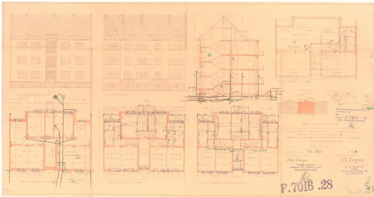
Il. 37 Ul. Tarnogajska. Elewacje i rzuty budynków nr 39, 1928, podpisano: Architekt: Hogreve (plik 124346). Archiwum Budowlane Wrocław, teczka 731.
