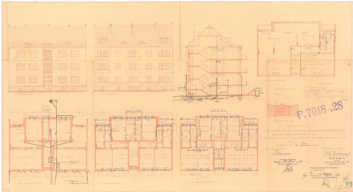
II. 39 Ul. Tarnogajska. Elewacji i rzuty budynku nr 43, 1928, podpisano: Architekt: Hogreve (plik 124361). Archiwum Budowlane Wrocław, teczka 731.
