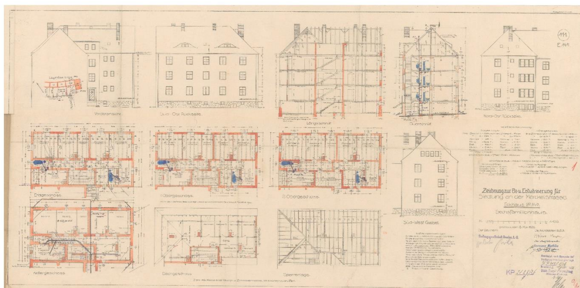
Il. 124 Ul. Sernicka. Plan sytuacyjny, rzuty, przekroje, elewacje sześciopiętrowego budynku narożnego nr 14, 1926, Inwestor: Siedlungsgesellschaft A. G., Architekci: Heim i Kempster, Wykonawca: Hermann Mathiba (plik 103614). Archiwum Budowlane Wrocław, teczka 3989
