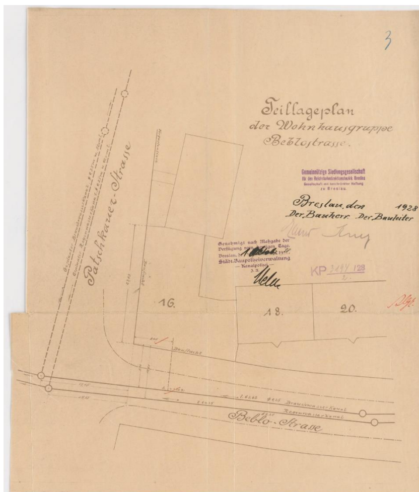
Il. 79 Ul. Jesionowa. Rzuty budynków 16, 18, 20, 1928, Inwestor: Gemeinnützige Siedlungsgesellschaft für den Reichsbahndirektionsbezirk Breslau (plik 97036). Archiwum Budowlane Wrocław, teczka 377.
