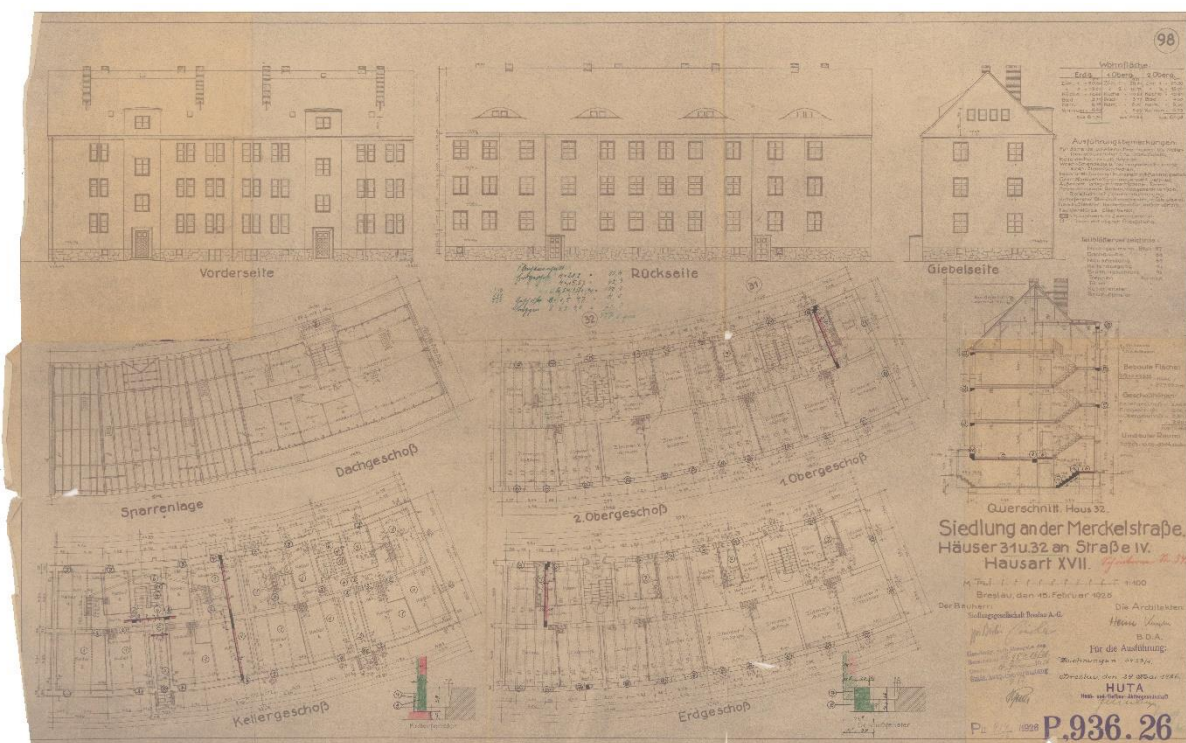
Il. 123 Ul. Sernicka. Rzuty, widoki elewacji budynku nr 31-32 (budynek typu 17), 1925, Inwestor: Siedlungsgesellschaft A. G., Architekci: Heim i Kempster, Wykonawca: HUTA Hoch- und Tiefbau-Aktionsgesellschaft, (plik 103619). Archiwum Budowlane Wrocław, teczka 3988.
