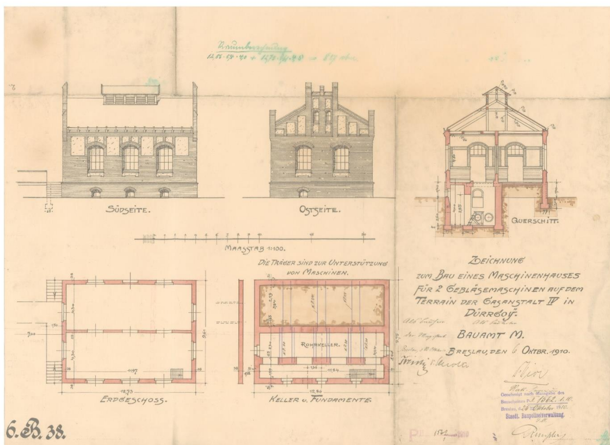
Il. 6 Gazownia. Maszynownia dla dwóch miechów gazowni nr IV, 1910, podpis nieczytelny (plik 127582). Archiwum Budowlane Wrocław,teczka 3456.
