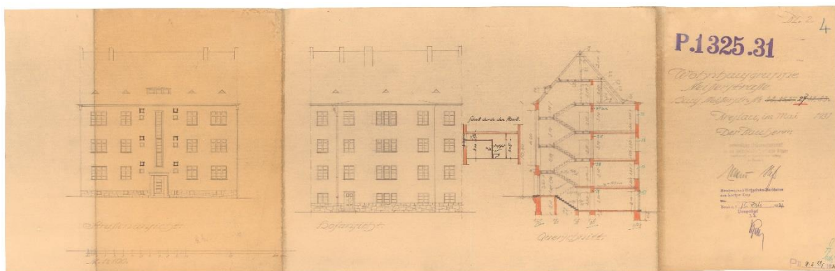
Il. 98 Ul. Nyska. Elewacje i przekrój budynku nr 27, 1931, Inwestor: Reichsbahn-Siedlungsgesellschaft Schlesien in Breslau (plik 103339). Archiwum Budowlane Wrocław, teczka 3090.
