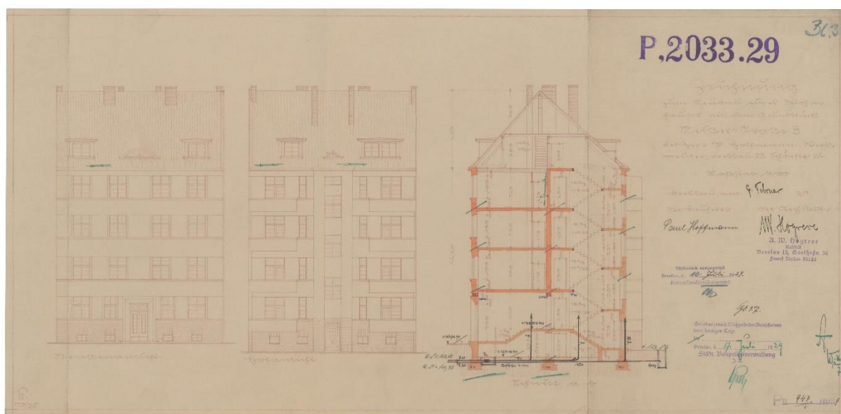
Il. 106 Ul. Nyska. Widoki elewacji i przekrój pięciokondygnacyjnego budynku, 1929, Architekt: August Wilhelm Hogreve (plik 103381). Archiwum Budowlane Wrocław, teczka 3091.
