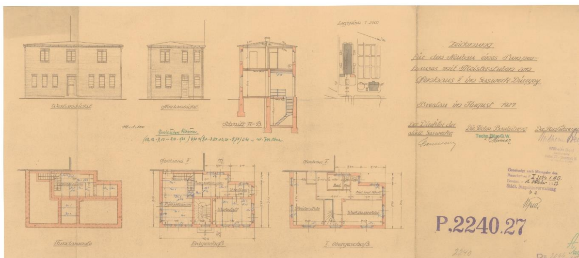
Il. 14 Gazownia. Pompownia i sterownia budynku piecowego, 1927, podpisano: Kierownik budowy: W. Beck (plik 127615). Archiwum Budowlane Wrocław, teczka 3456.
