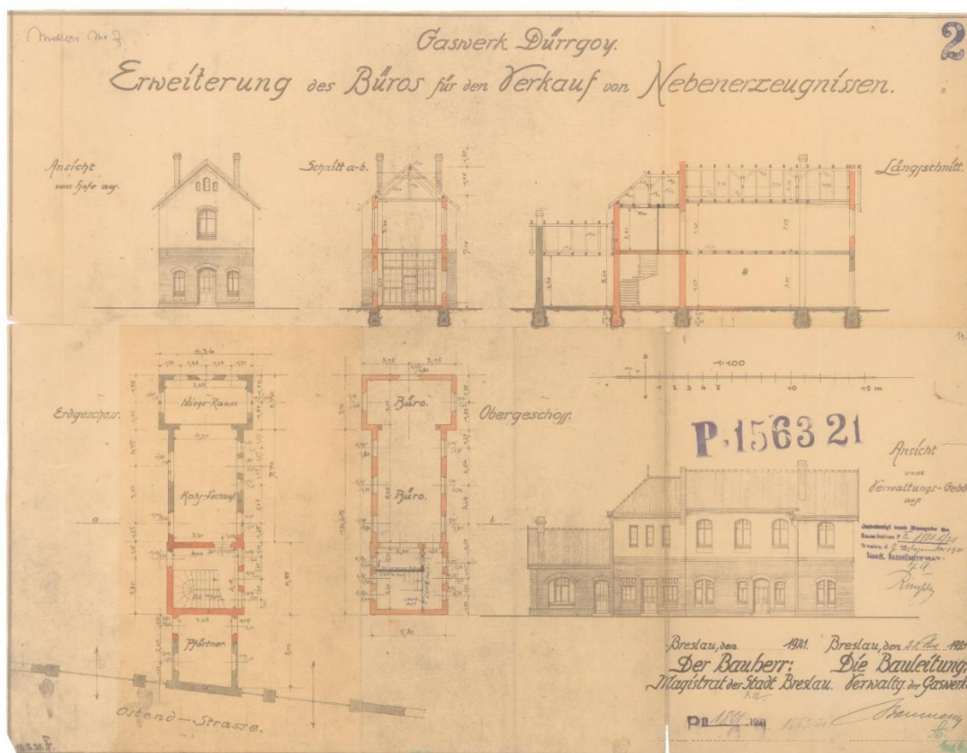
Il. 11 Gazownia. Rozbudowa budynku biurowego i budynku sprzedaży, 1921, podpisano: Magistrat: Rimpler (plik 127594). Archiwum Budowlane Wrocław,teczka 3456.
