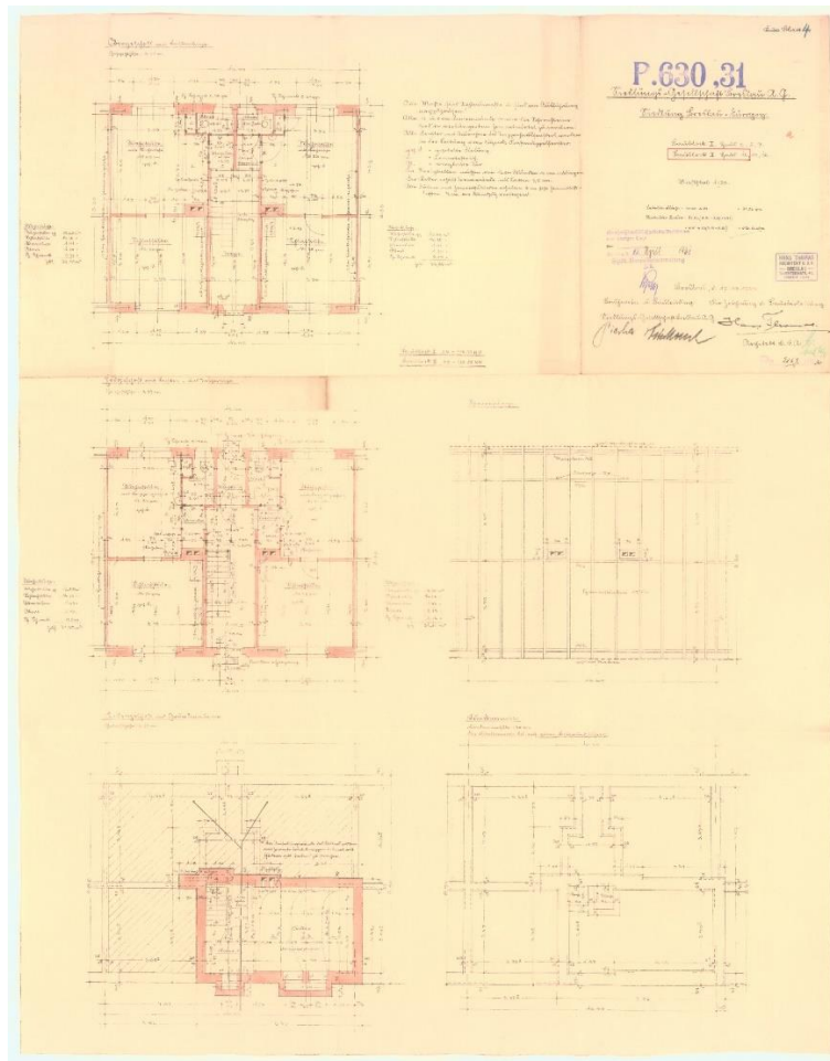
II. 59 Ul. Złotostocka. Projekt budynku przy ul. Złotostockiej 12, 1931, wznoszonego przez Siedlung Gesellschaft Breslau A. G., podpisano: Architekt: Hans Thomas (plik 124474). Archiwum Budowlane Wrocław,teczka 3648.
