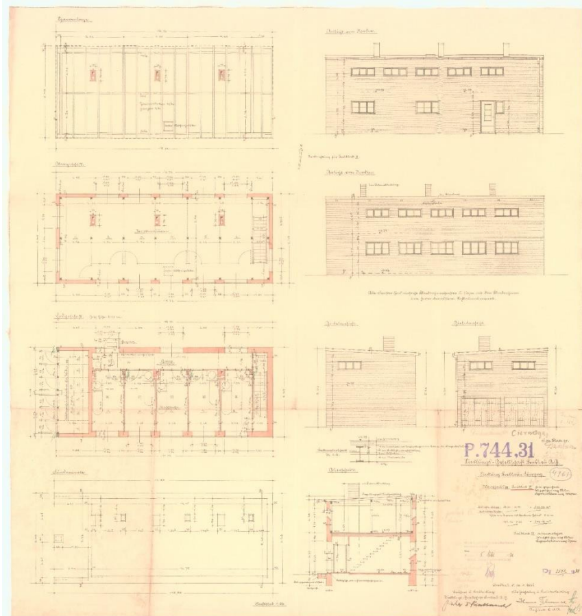
Il. 61 Ul. Złotostocka. Rzut sytuacyjny łaźni i ustępów, 1931, podpisano: Architekt: Hans Thomas (plik 124486). Archiwum Budowlane Wrocław, teczka 3648.
