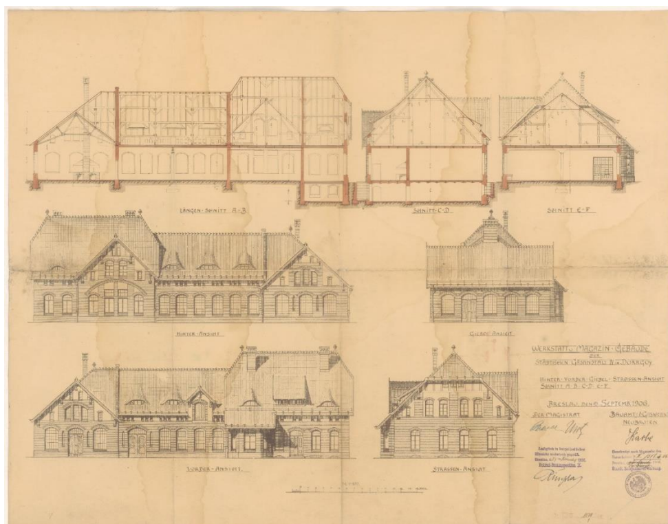
Il. 1 Gazownia. Budynek warsztatowy i magazynowy, 1906, podpisano: Urząd Budowlany: Karbe, Magistrat: Wirtz, (plik 127560). Archiwum Budowlane Wrocław,teczka 3455.
