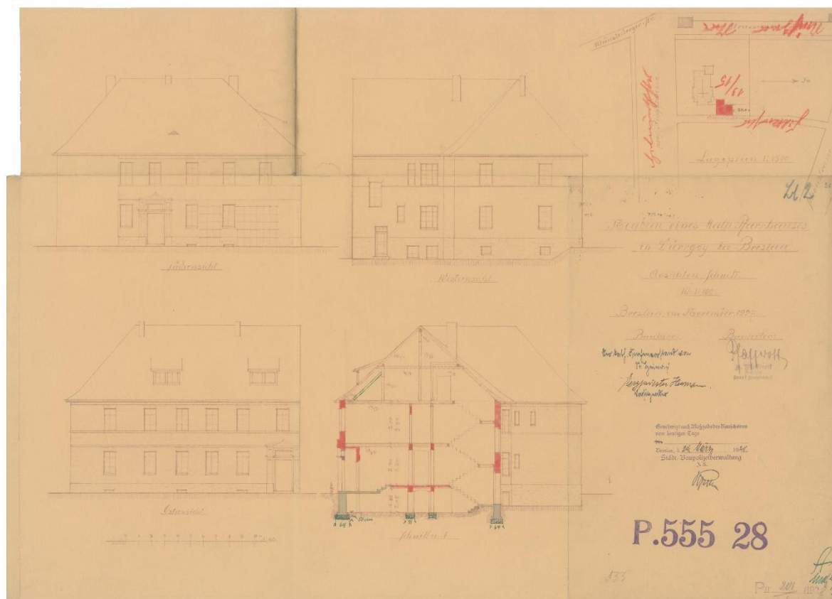
II. 88 Ul. Nowokościelna. Widoki elewacji plebanii przy nowym kościele katolickim pw. Świętego Ducha, 1928, Architekt: B. Pfafferott (plik 175831). Archiwum Budowlane Wrocław, teczka 878.
