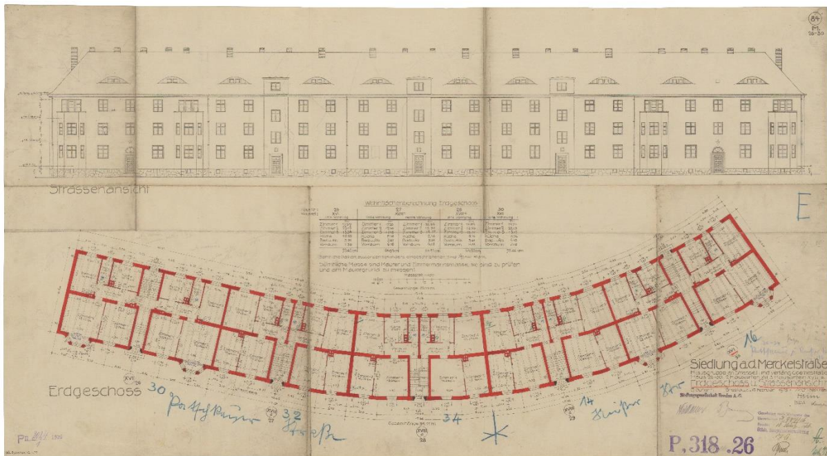
Il. 115 Ul. Paczkowska. Rzuty i widoki elewacji budynków 26-30, Inwestor: Siedlungsgesellschaft Breslau A. G., Architekt: Paul Heim (plik 103253). Archiwum Budowlane Wrocław, teczka 3517
