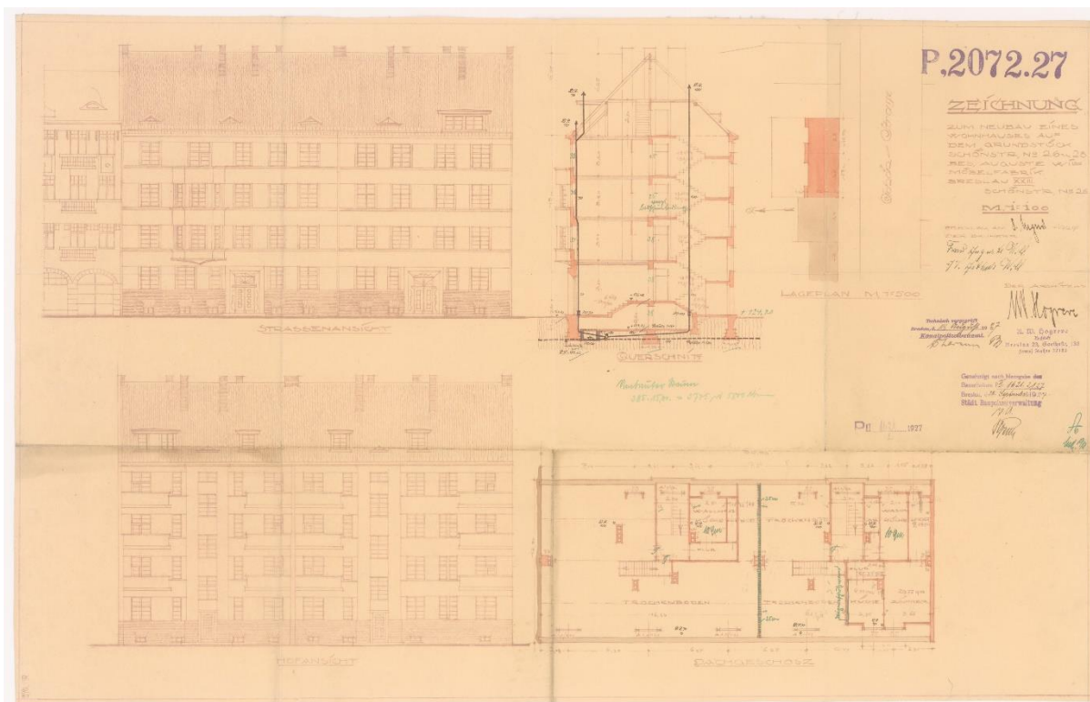
Il. 118 Ul. Piękna. Elewacje, rzut i przekrój budynku nr 26-28, 1927, Inwestor: Auguste Will, Architekt: August Wilhelm Hogueve (plik 103163). Archiwum Budowlane Wrocław, teczka 3980
