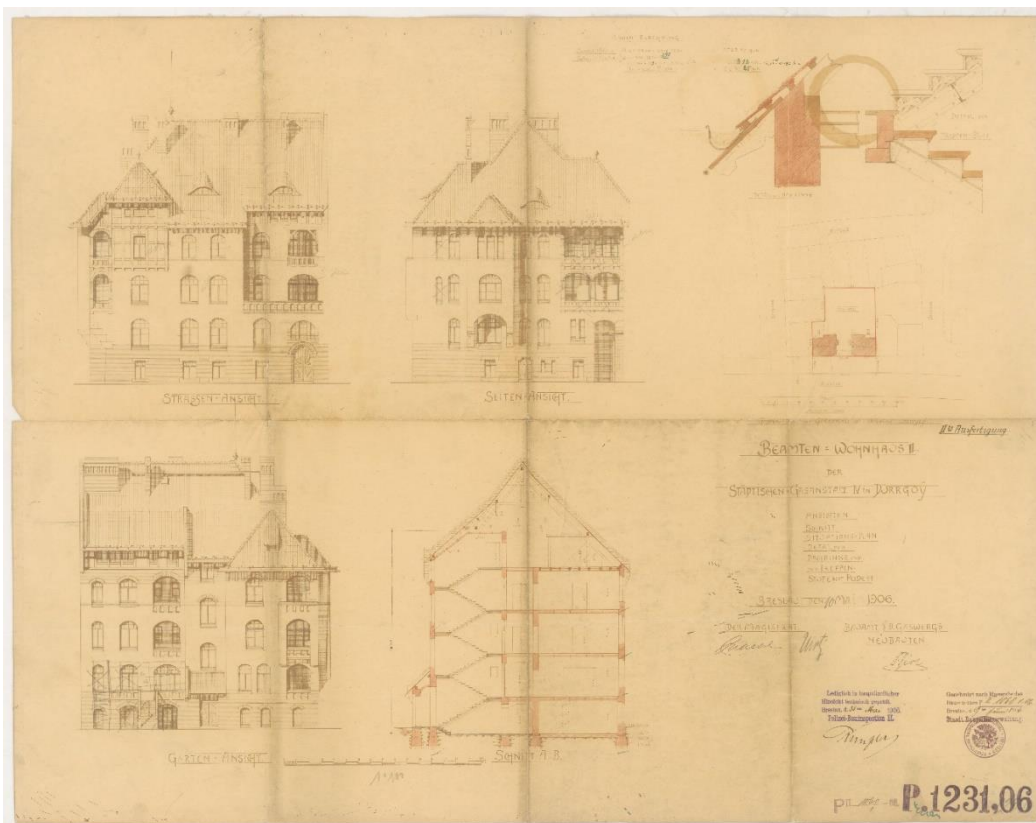
Il. 27 Ul. Gazowa. Plan budynku nr 2 dla urzędników gazowni, 1906, podpisano: Magistrat i Biuro Gazowni: Wirtz (plik 157367). Archiwum Budowlane Wrocław, teczka 3458.
