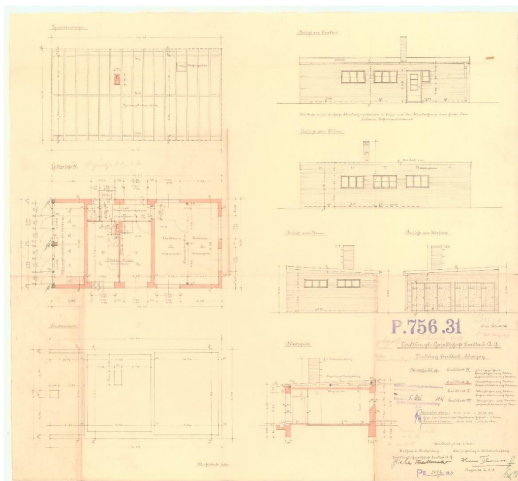
Il. 56 Ul. Złotostocka. Budynek 6-12 wznoszony przez Siedlung Gesellschaft Breslau A. G., podpisano: Architekt: Hans Thomas (plik 124468). Archiwum Budowlane Wrocław, teczka 3648.
