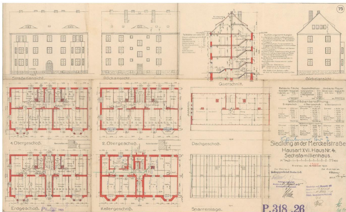
Il. 121 Ul. Sernicka. Budynek sześciorodzinny nr 4, 1925, Inwestor: Siedlungsgesellschaft A. G., Architekci: Heim i Kempster (plik 103583). Archiwum Budowlane Wrocław, teczka 3988.
