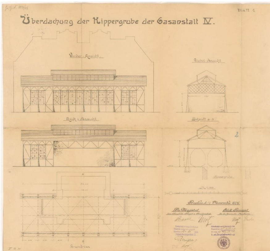
Il. 2 Gazownia. Projekt zadaszenia rampy rozładowniczej, 1906, podpisano: Urząd Budowlany: Karbe, Magistrat: Wirtz, Archiwum Budowlane Wrocław (plik 127566). Archiwum Budowlane Wrocław,teczka 3455.
