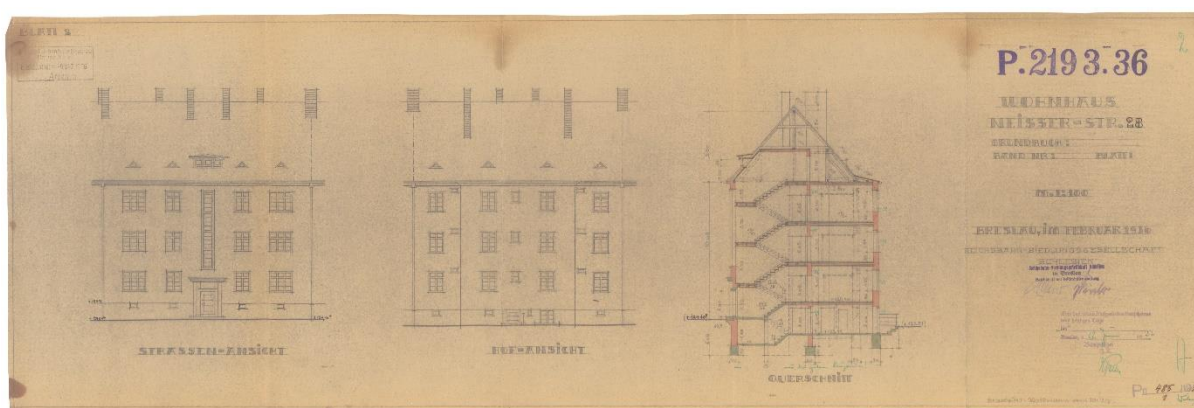
Il. 99 Ul. Nyska. Elewacje i przekrój budynku nr 28, 1936, Inwestor: Reichsbahn-Siedlungsgesellschaft Schlesien in Breslau (plik 103346). Archiwum Budowlane Wrocław, teczka 3090.
