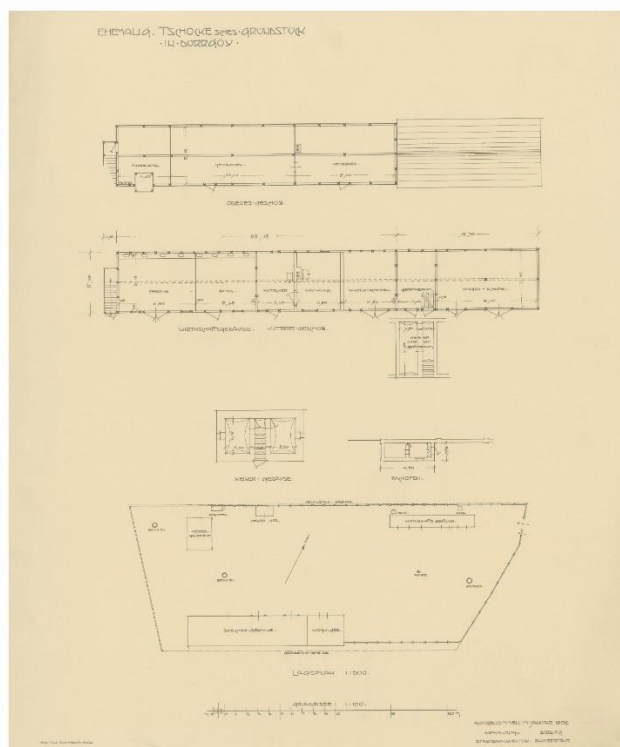
Il. 30 Dawne gospodarstwo Tschocke na Tarnogaju. Rzut stajni i obór oraz stodół w górnej kondygnacji, w dolnej partii plan założenia, 1902 (plik TP424, sygn. 8631).
