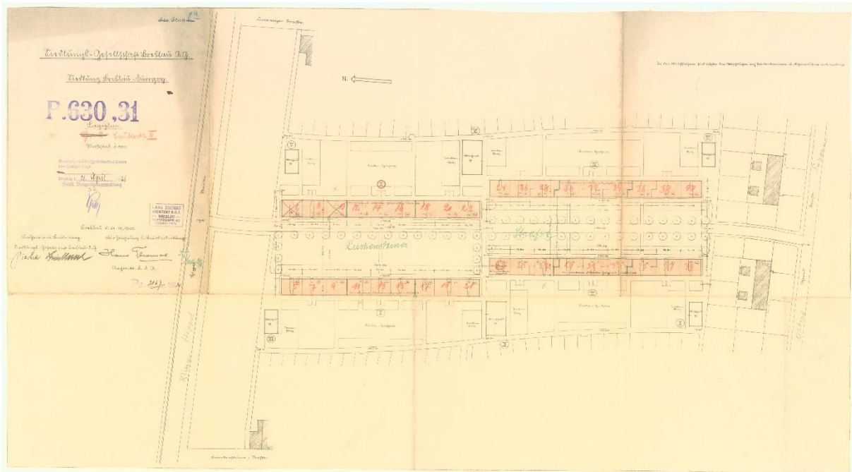
Il. 57 Ul. Złotostocka. Plan sytuacyjny zabudowy ul. Złotostockiej wraz z zielenią, 1930, podpisano: Architekt: Hans Thomas (plik 124470). Archiwum Budowlane Wrocław,teczka 3648.
