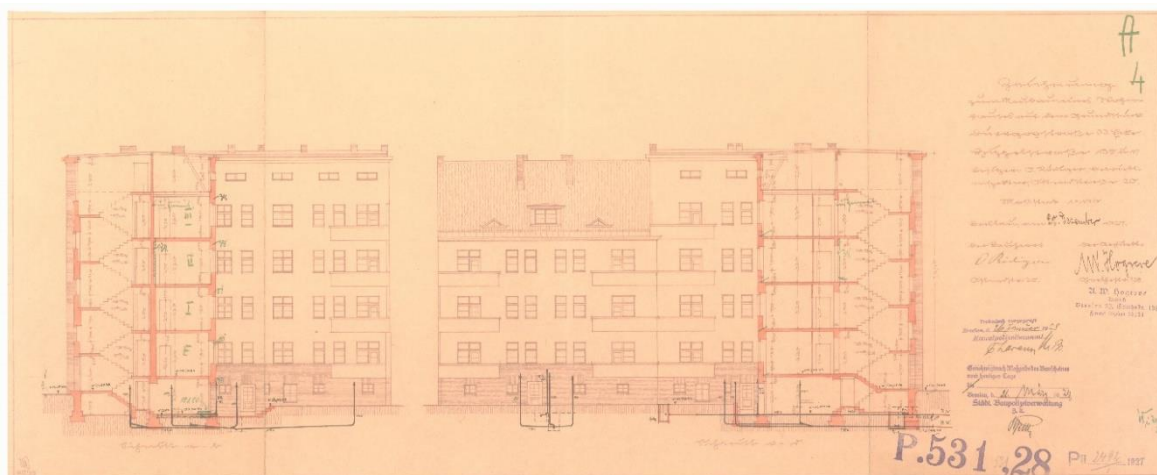
Il. 34 Ul. Tarnogajska. Elewacji i przekroje budynków nr 15-17, 1927, podpisano: Architekt: Hogreve (plik 124315). Archiwum Budowlane Wrocław,teczka 731.
