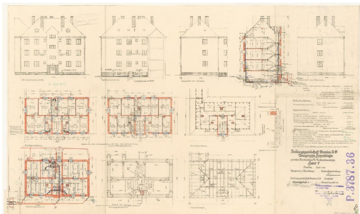
Il. 44 Ul. Ząbkowicka. Rzuty i przekroje budynków wybudowanych przez Siedlung Gesellschaft Breslau A. G. między ulicami Ząbkowicką i Złotostocką, 1936 (plik 124603). Archiwum Budowlane Wrocław,teczka 1105.
