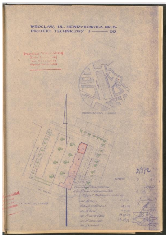
Il. 76 Ul. Henrykowska. Rzut sytuacyjny ulicy z zaznaczoną zielenią, 1952, Inwestor: Prezydium Wojewódzkiej Rady Narodowej. Wydział Budownictwa, Architekt: Marian Broś, tech. Zbigniew Kotulewicz, inż. Stanisław Tokarowski, inż. J. Kruhlik (plik 8 rys. 1). Archiwum Budowlane Wrocław, DPL 50.
