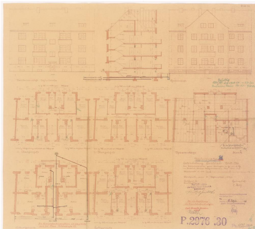
Il. 120 Ul. Piękna. Widok elewacji, rzuty i przekroje budynku nr 29, 1930, Inwestor: Postheimstätte gem. Baugenossenschaft G. m. b. H. Breslau, Architekt: Wolf, Wykonawca: Carl Brandt (plik 103178). Archiwum Budowlane Wrocław, teczka 3980.
