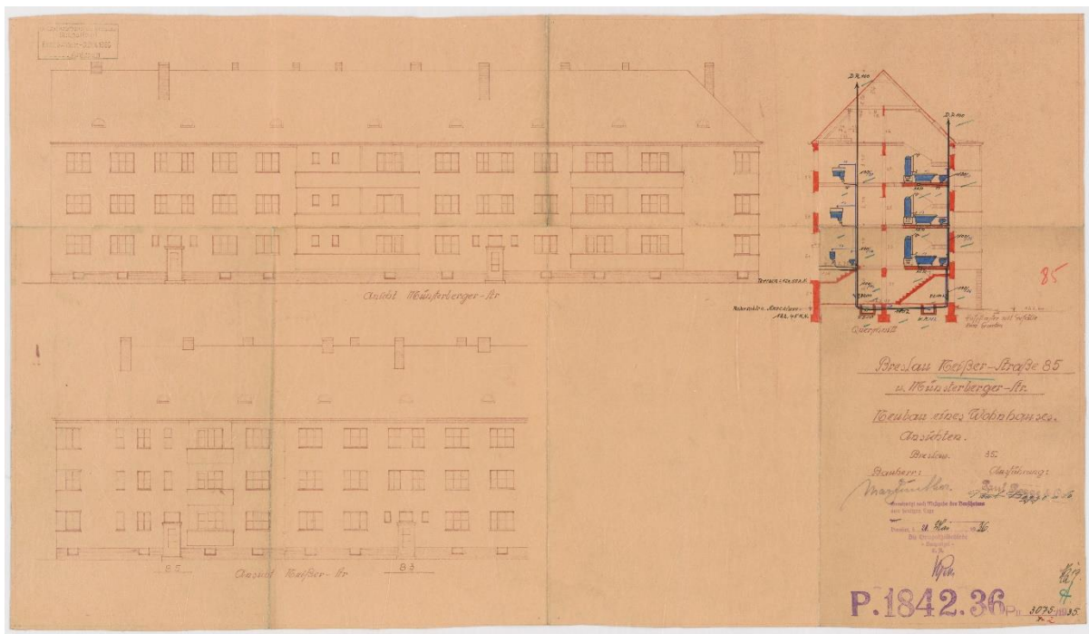
Il. 113 Ul. Nyska. Narożny budynek przy ul. Nyskiej i Ziębickiej, widoki elewacji i przekrój, 1935, Realizacja: Paul Rogge & Co (plik 198886). Archiwum Budowlane Wrocław,teczka 3093.
