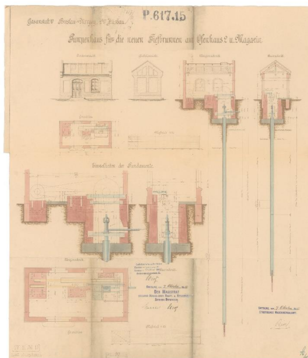
Il. 9 Gazownia. Pompa dla studni głębinowej drugiego pieca i magazynu, 1915, podpisano: Magistrat: Wirtz (plik 127587). Archiwum Budowlane Wrocław, teczka 3456.
