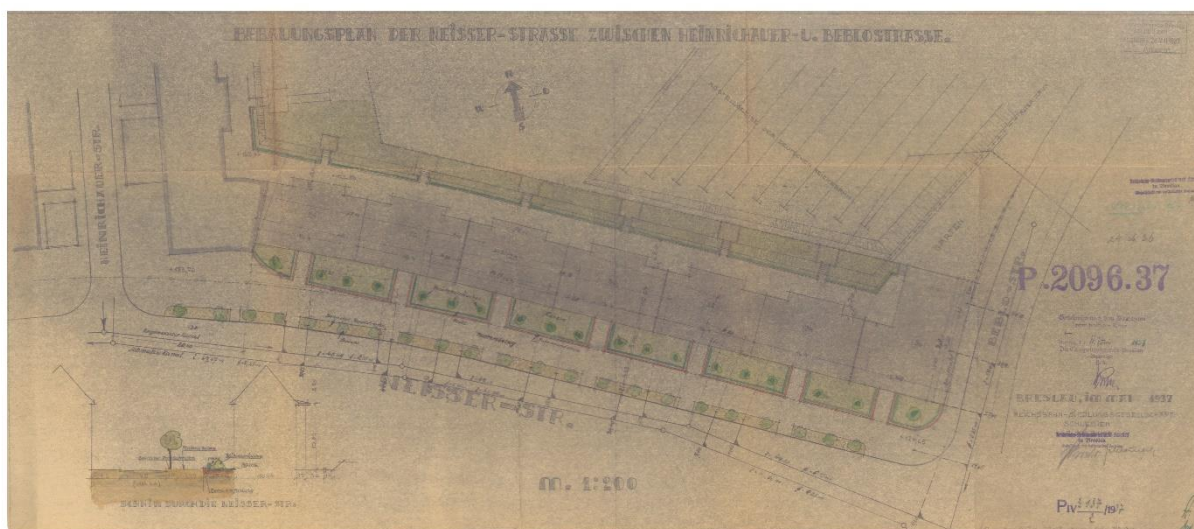
Il. 94 Ul. Nyska. Plan sytuacyjny budynków między ulicami Nyską i Jesionową z zaznaczeniem przedogródków, 1937, Inwestor: Reichsbahn-Siedlungsgesellschaft Schlesien in Breslau (plik 103320). Archiwum Budowlane Wrocław,teczka 3089.
