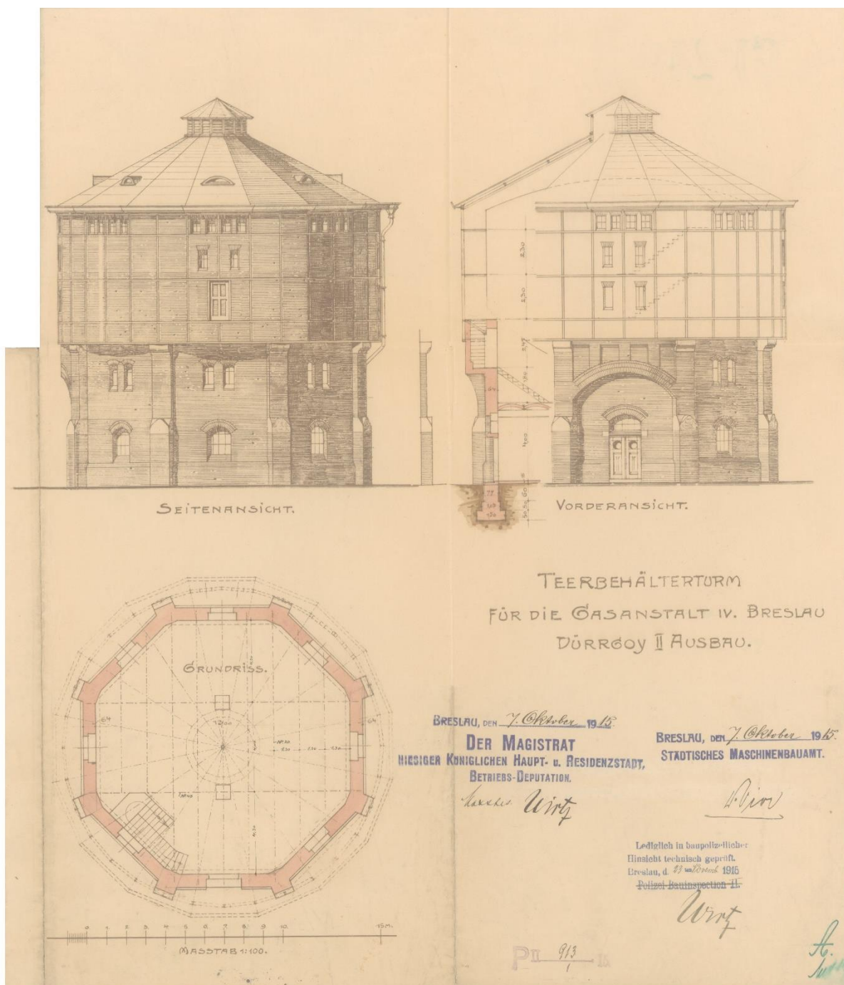
Il. 7 Gazownia. Zbiornik na smołę – druga rozbudowa, 1915, podpisano: Urząd Budowlany: podpis nieczytelny, Magistrat: Wirtz (plik 127584). Archiwum Budowlane Wrocław,teczka 3456.
