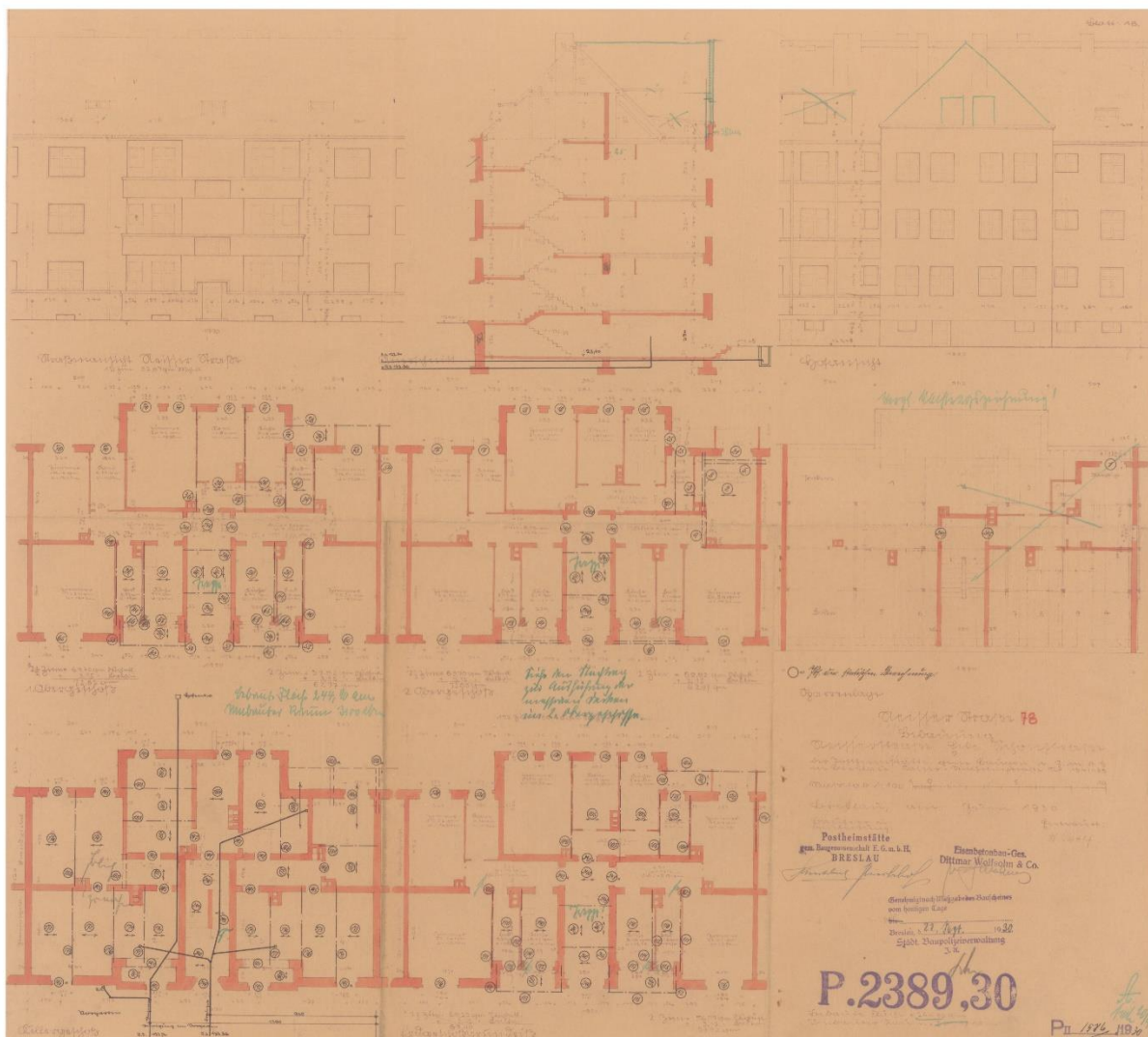
Il. 111 Ul. Nyska. Rzuty i elewacje budynku nr 78, 1930, Inwestor: Postheimstätte gem. Baugenossenschaft G. m. b. H. Breslau, Wykonawca: Eisenbetonbau-Gesellschaft Dittmar Wolfsohn & Co. (plik 103206). Archiwum Budowlane Wrocław, teczka 3093.
