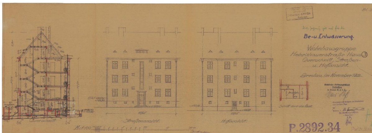
Il. 71 Ul. Henrykowska. Szkice kanalizacyjne budynku nr 3, 1933, Inwestor: Reichsbahn-Siedlungsgesellschaft Schlesien in Breslau, Przedsiębiorca: Richard Aust und Co (plik 103482). Archiwum Budowlane Wrocław,teczka 1711.
