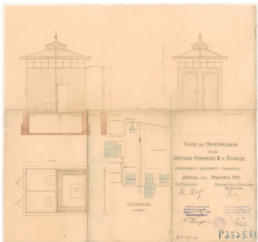
Il. 5 Gazownia. Pisuar i szalety, 1907, podpisano: Urząd Budowlany: Karbe, Magistrat: Wirtz (plik 127579). Archiwum Budowlane Wrocław,teczka 3455.
