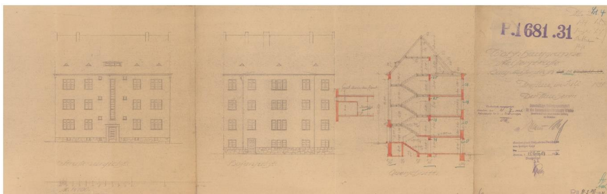
Il. 95 Ul. Nyska. Widoki elewacji i przekrój budynku nr 25, 1931, Inwestor: Reichsbahn-Siedlungsgesellschaft Schlesien in Breslau (plik 103323). Archiwum Budowlane Wrocław,teczka 3089.
