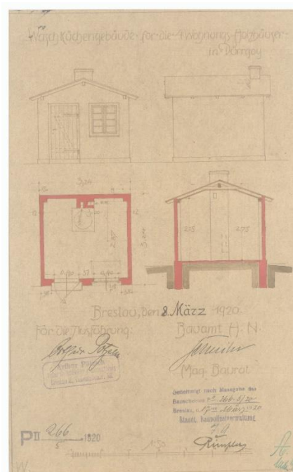
Il. 24 Ul. Gazowa. Pralnie dla czterech mieszkań, 1920, podpisano: Magistrat: Rimpler, Architekt: Pötsch (plik 157347). Archiwum Budowlane Wrocław, teczka 3458.
