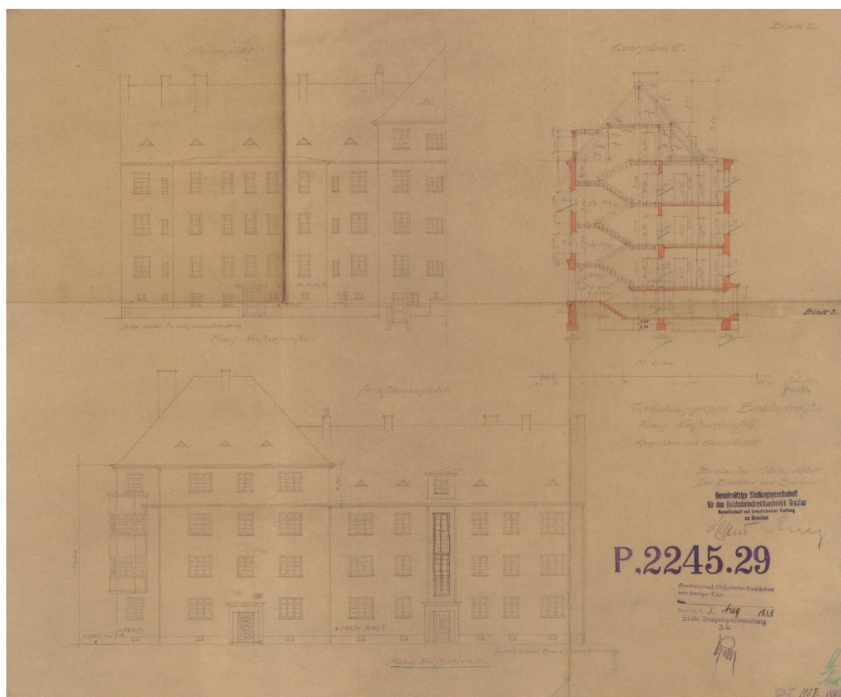
Il. 102 Ul. Nyska. Elewacje i przekrój budynku narożnego przy ul. Nyskiej i Jesionowej, 1929, Inwestor: Gemeinnützige Siedlungsgesellschaft für den Reichsbahndirektionsbezirk Breslau (plik 97020). Archiwum Budowlane Wrocław, teczka 3091.
