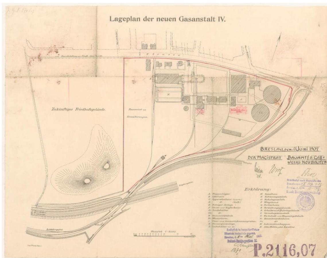
Il. 4 Gazownia. Plan sytuacyjny nowej gazowni IV, 1907, podpisano: Urząd Budowlany: podpis nieczytelny, Magistrat: Wirtz (plik 127575). Archiwum Budowlane Wrocław, teczka 3455.
