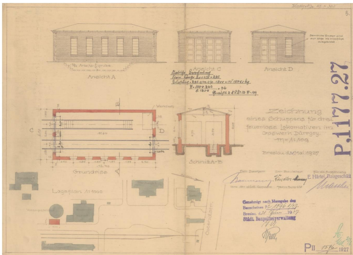
Il. 13 Gazownia. Szopa dla trzech bezogniowych lokomotyw, 1927, podpisano: Kierownik budowy: Kindler, Wykonawca: E. Härtel (plik 127614). Archiwum Budowlane Wrocław, teczka 3456.
