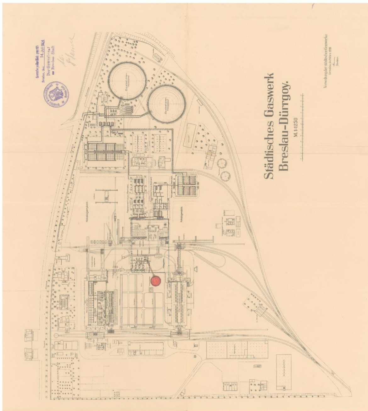
Il. 18 Gazownia. Plan sytuacyjny z rysunkiem instalacji technicznej, 1929 (plik 127632). Archiwum Budowlane Wrocław,teczka 3456.
