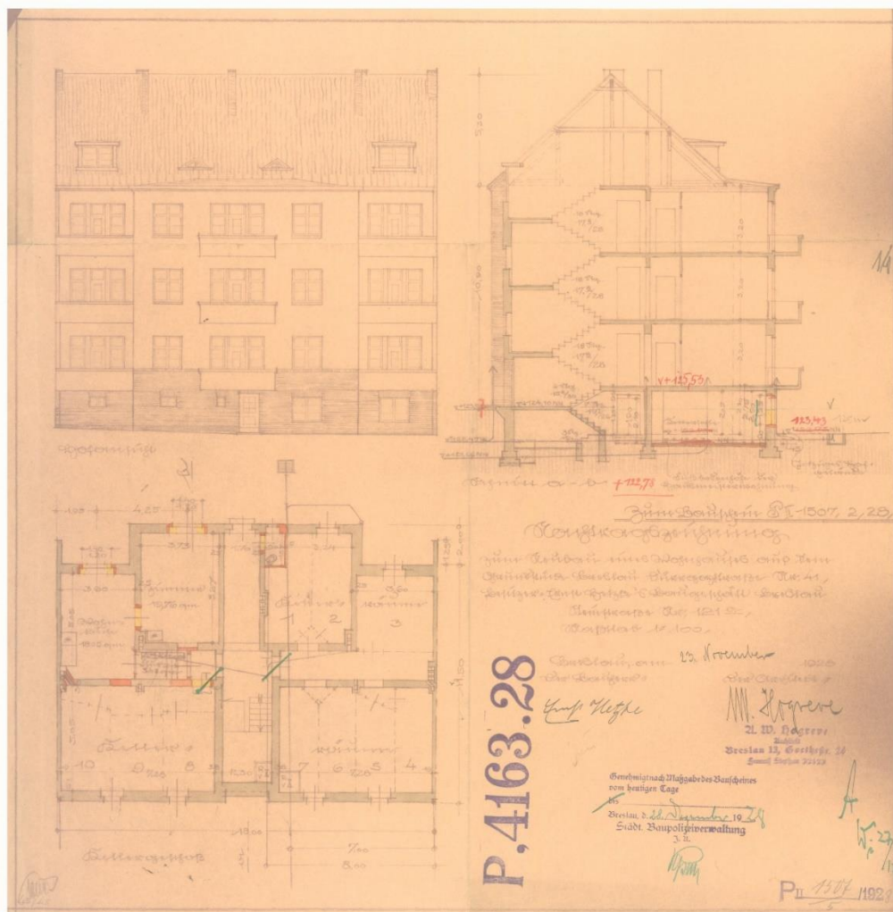
Il. 38 Ul. Tarnogajska. Elewacje i rzuty budynku nr 41, 1928, podpisano: Architekt: Hogreve (plik 124358). Archiwum Budowlane Wrocław, teczka 731.
