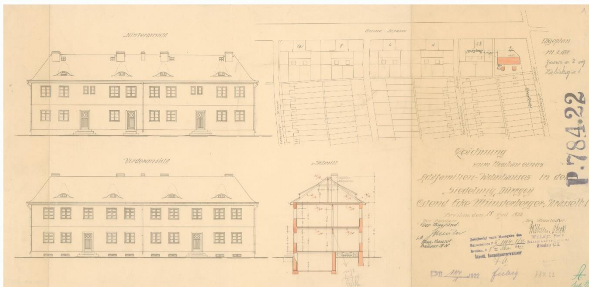
Il. 22 Ul. Gazowa. Niezachowany budynek na narożniku ulic Gazowej i Ziębickiej, 1922, podpisano: Kierownik budowy: Wilhelm Beck, radca murarski Breslau 13 (plik 157339). Archiwum Budowlane Wrocław, teczka 3458.
