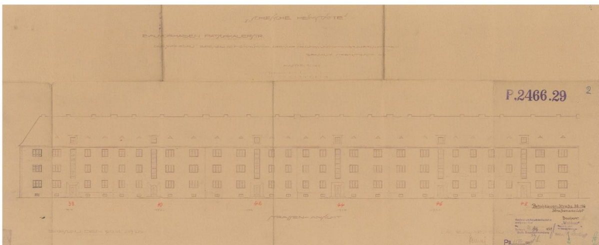
Il. 116 Ul. Paczkowska. Elewacja uliczna budynków 38-46, 1929, Inwestor: „Der Wohnbau” Breslau Gemeinnützige Schlesische Siedlungs- und Wohnungsbaugesellschaft M. B. H., Schlesische Heimstätte (plik 103266). Archiwum Budowlane Wrocław, teczka 3518
