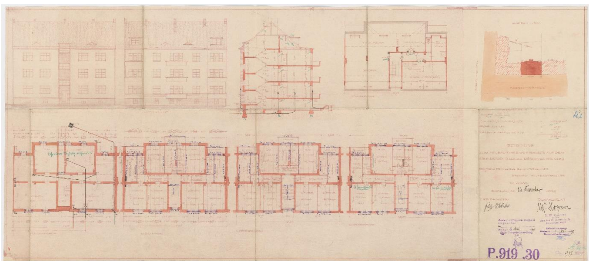
II. 40 Ul. Tarnogajska. Elewacje i rzuty budynku nr 59, 1929, podpisano: Architekt: Hogreve (plik 124437). Archiwum Budowlane Wrocław, teczka 733.
