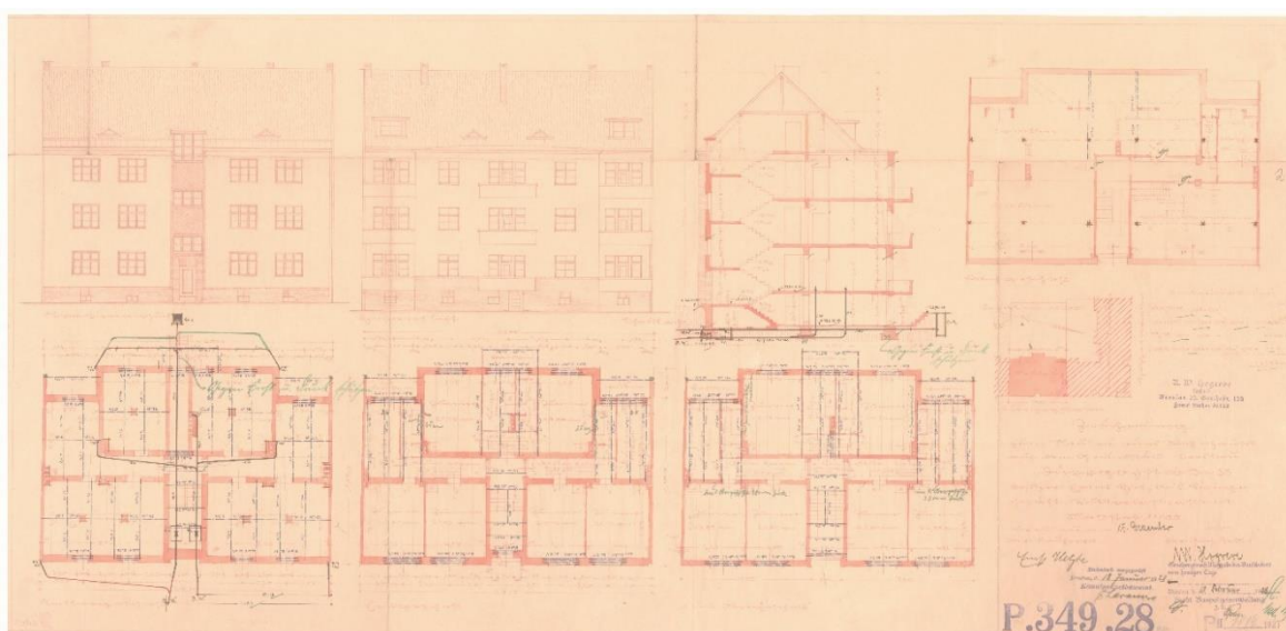
Il. 36 Ul. Tarnogajska. Elewacje i rzuty budynku nr 35, 1927, podpisano: Architekt: Hogreve (plik 124330). Archiwum Budowlane Wrocław,teczka 731.
