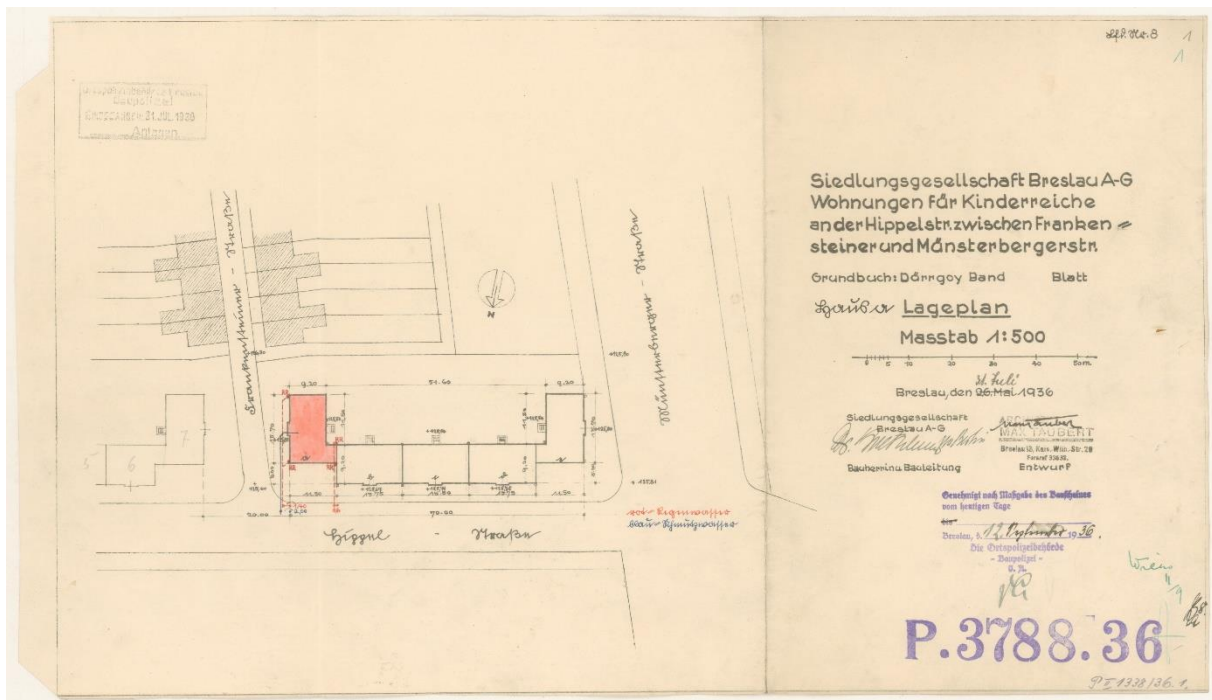
Il. 43 Ul. Ząbkowicka. Plan sytuacyjny budynku wybudowany przez Siedlung Gesellschaft Breslau A. G., narożnik ulic Ząbkowickiej i Klimasa, 1936, podpisano: Projekt: Max Taubert (plik 124599). Archiwum Budowlane Wrocław,teczka 1105.
