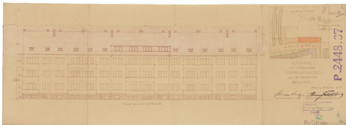
Il. 81 Ul. Jesionowa. Widok elewacji ogrodowej budynku wielorodzinnego, 1937 (plik 97037). Archiwum Budowlane Wrocław, teczka 377.
