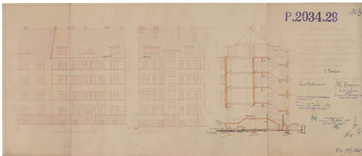
Il. 107 Ul. Nyska. Widoki elewacji i przekrój pięciokondygnacyjnego budynku, 1929, Architekt: August Wilhelm Högrevé (plik 103391). Archiwum Budowlane Wrocław,teczka 3091.
