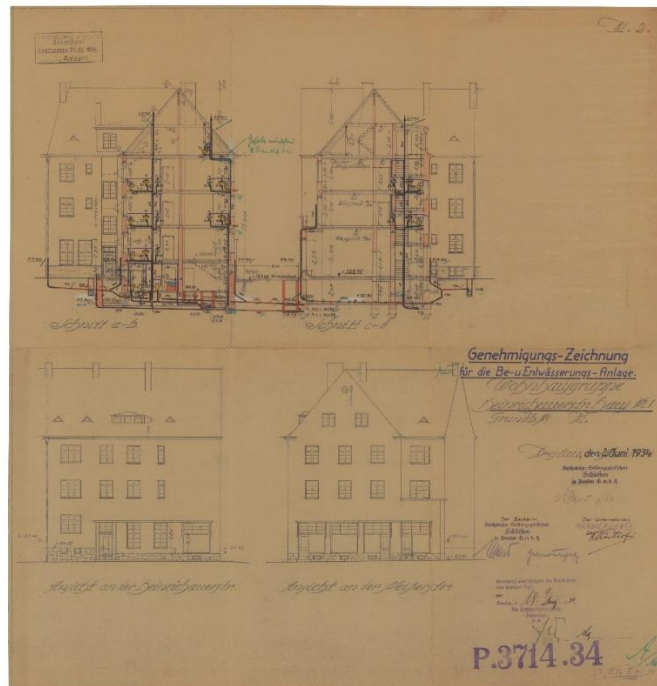
Il. 63 Ul. Henrykowska. Przekroje i rysunki elewacji budynku nr 1, 1934, Inwestor: Reichsbahn-Siedlungsgesellschaft Schlesien in Breslau, Przedsiębiorca: Richard Aust und Co. (plik 103442). Archiwum Budowlane Wrocław, teczka 1711.
