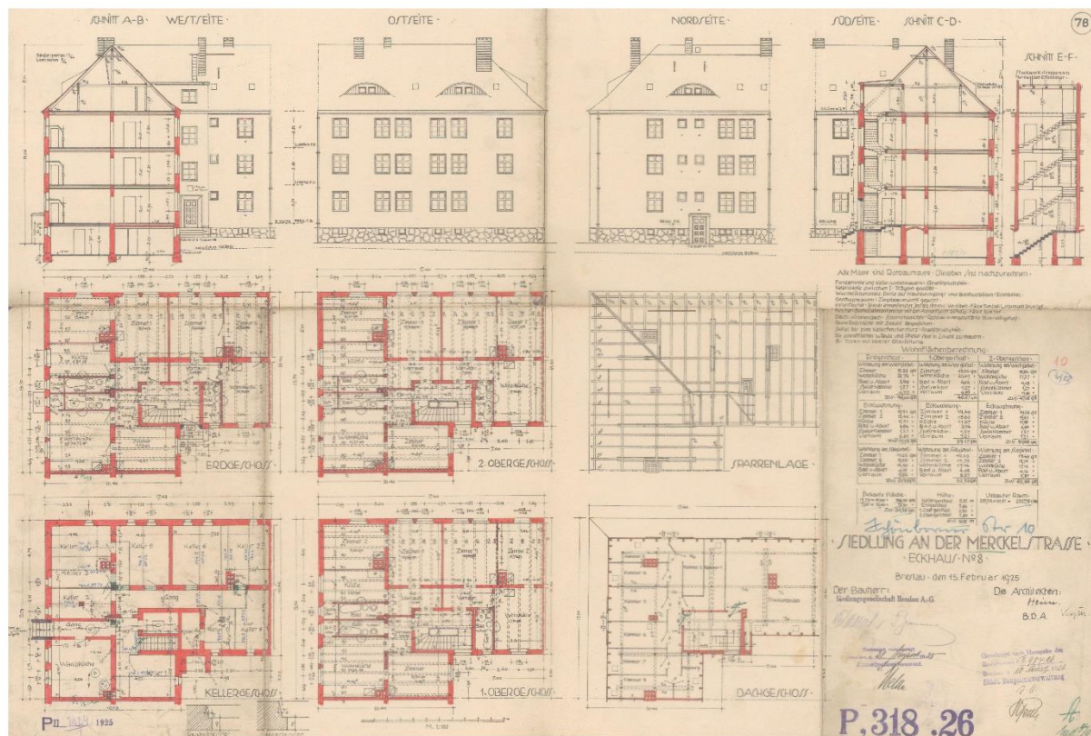
Il. 122 Ul. Sernicka. Przekrój, widoki elewacji domu narożnego nr 8, 1925, Inwestor: Siedlungsgesellschaft A. G., Architekci: Heim i Kempster (plik 103600). Archiwum Budowlane Wrocław, teczka 3988.
