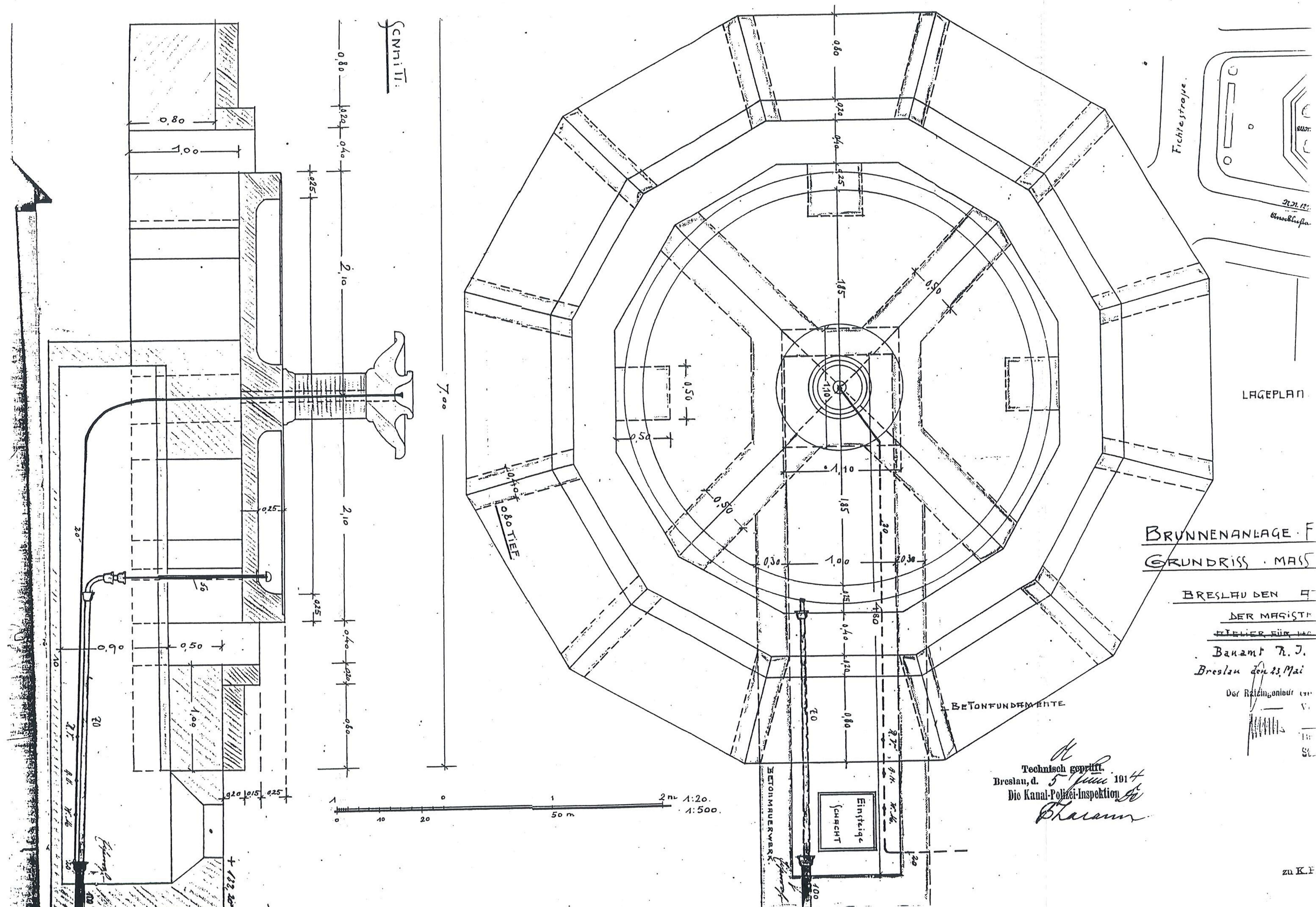
21. Projekt fontanny i plan sytuacyjny jej lokalizacji na skwerze przy ul. Przestrzennej. 1914.
