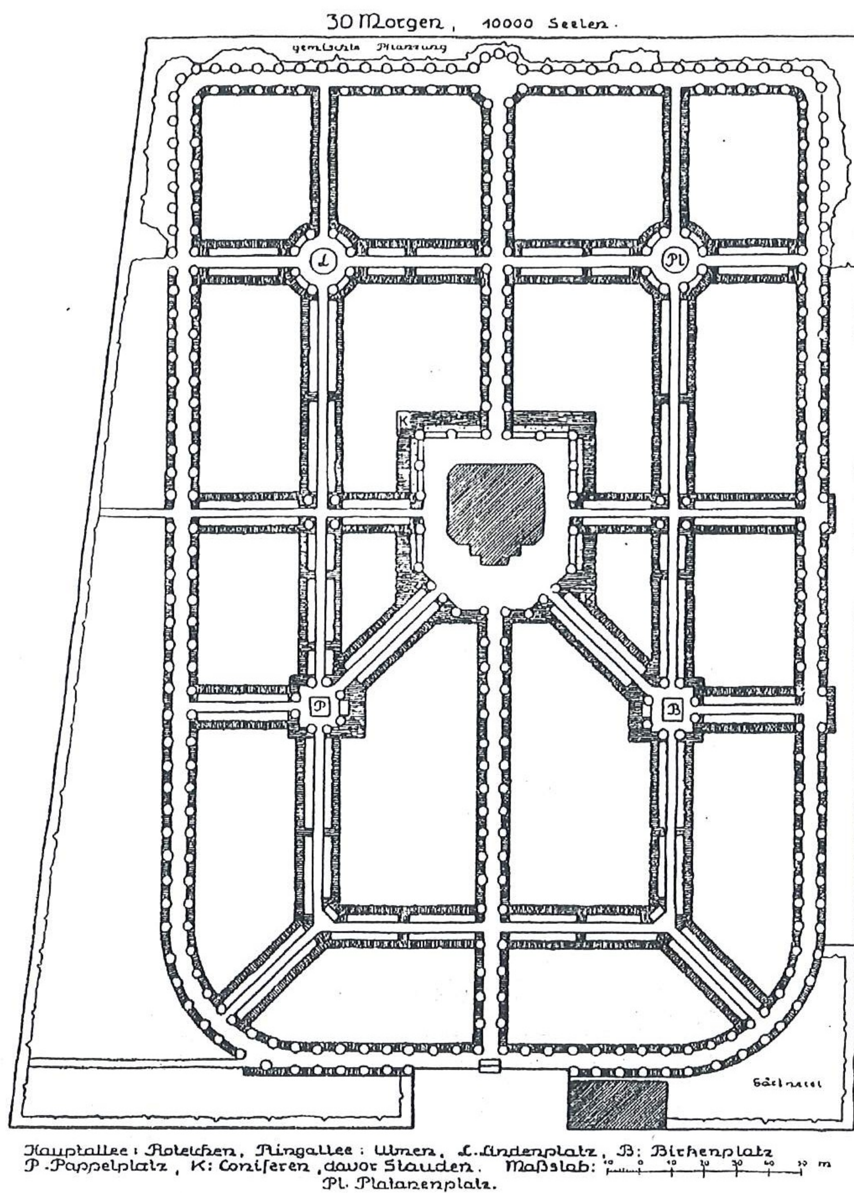
Plan einer Friedhofsanlage für eine größere Gemeinde.
