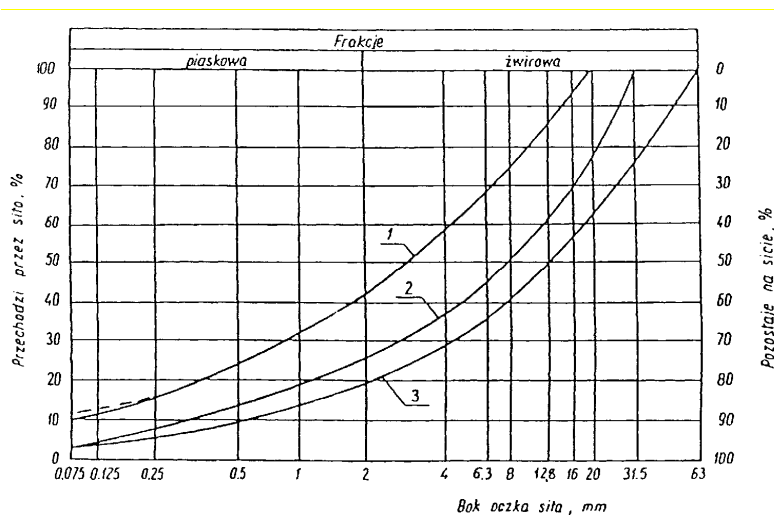
Rysunek 1. Pole dobrego uziarnienia kruszyw przeznaczonych na podbudowy wyk. metodą stabilizacji mechanicznej
